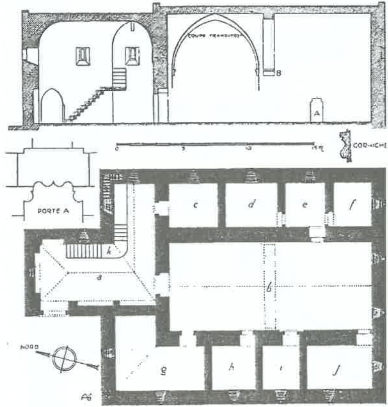
Plan-5: HAYTAR BEY KÖŞKÜ (Gabriel'den)
