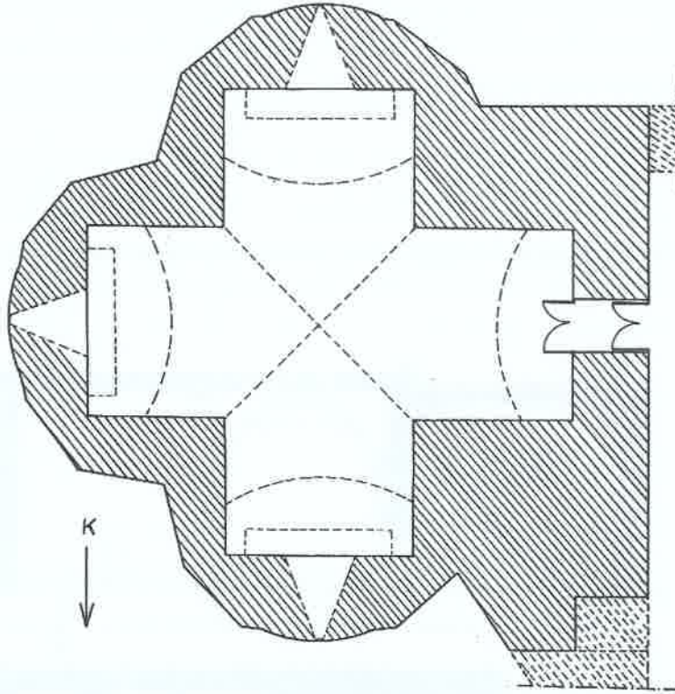
Plan-3: OK BURCU ZEMİN KAT PLANI ölçek:1/200
