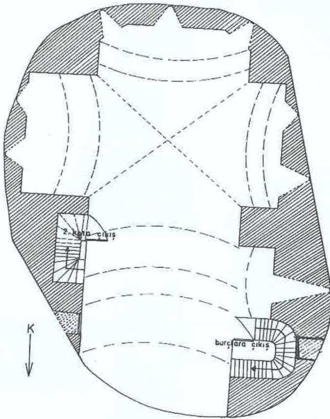
Plan-1: YOĞUN BURÇ 2. KAT PLANI ölçek: 1/200
