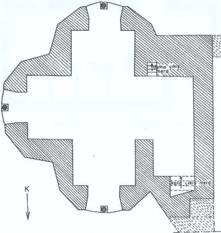
Plan-4: OK BURCU 2. KAT PLANI ölçek:1/200
