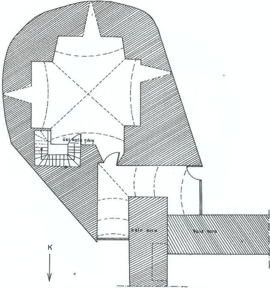
Plan-2: YOĞUN BURÇ ZEMİN KAT PLANI ölçek 1/200
