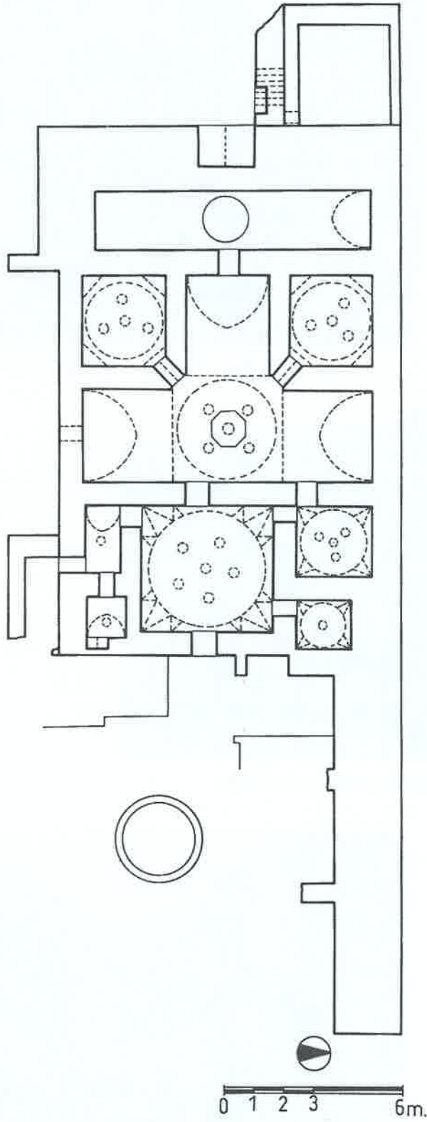
Lev. 2: Balta Bey Hamamı, rölöve planı.
