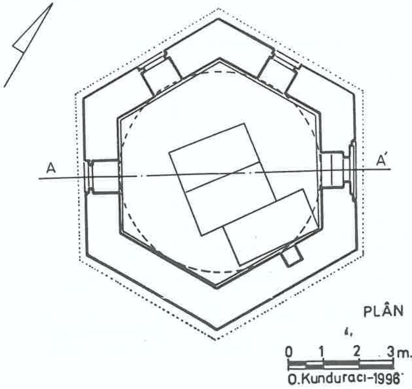
Çizim 1: Konya Güneysınır İlçesi Gürağaç Köyü Aktürbe Tekkesi Kesit-Plan
