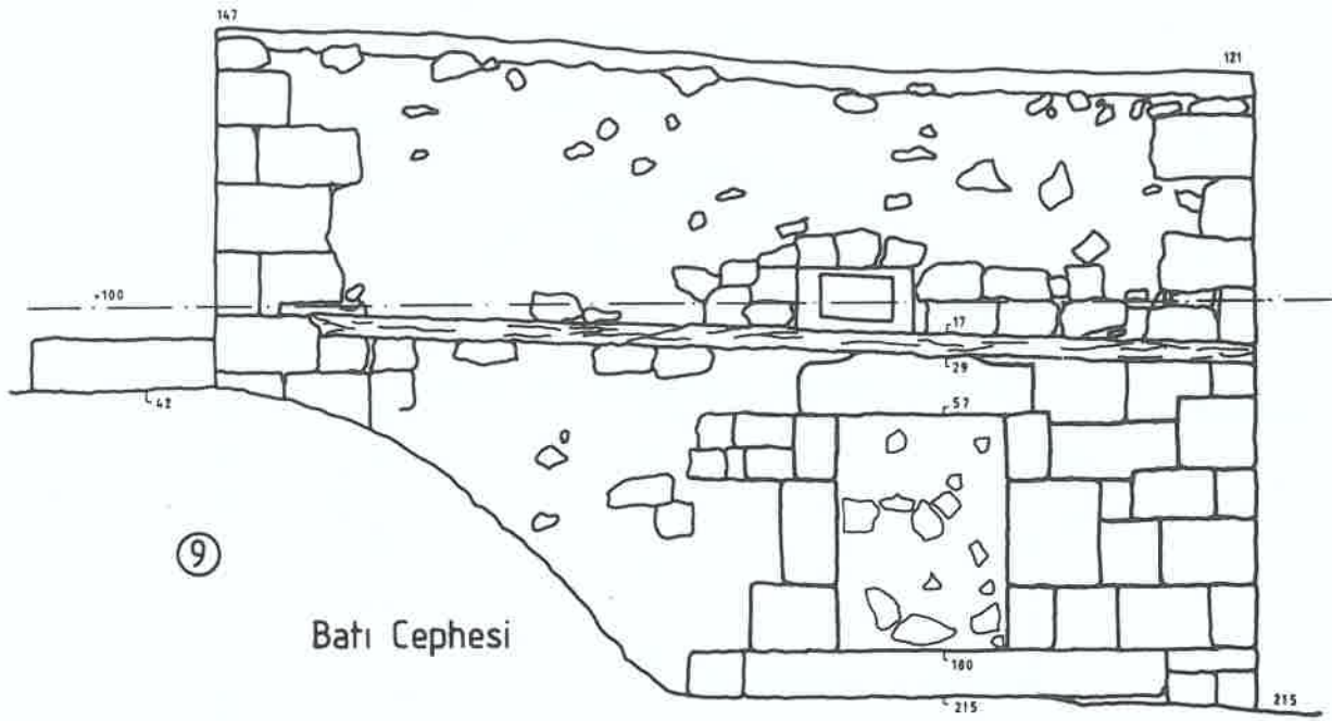
Niğde-Güllüce Köyü ŞEYH İBRAHİM TEKKESİ'NİN TÜRBEŞİ Röleve - Çizim: Halit Çal
