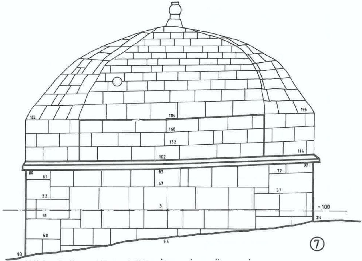
Niğde-Güllüce Köyü ŞEYH İBRAHİM KÜMBETİ
