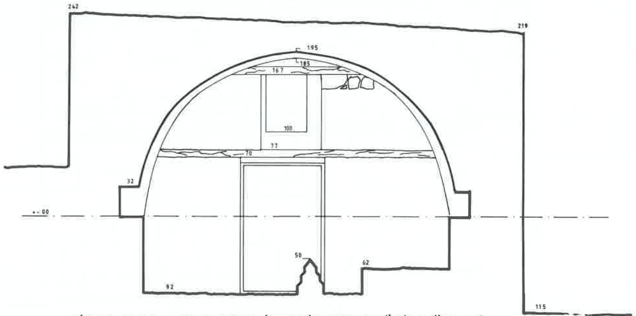
NİĞDE - Güllüce Köyü, ŞEYH İBRAHİM TEKKESİ'NİN TÜRRESİ
