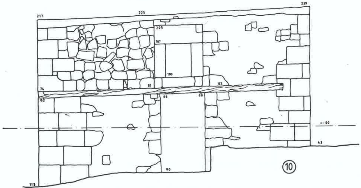
Niğde Güllüce Köyü ŞEYH İBRAHİM TEKKESİ'NİN TÜRBEŞİ Röleve Çizim: Halit Çal
