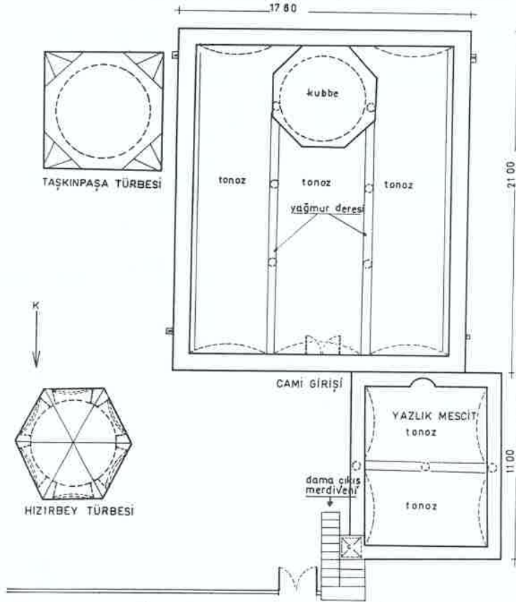
NEVŞEHİR ÜRGÜP TAŞKINPAŞA CAMİ PLANI
