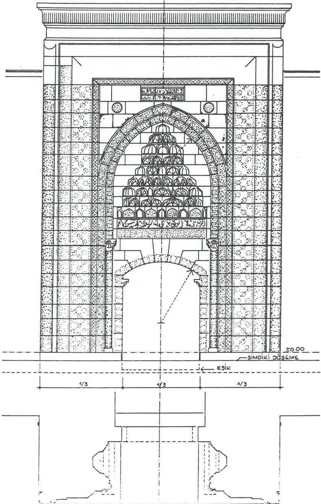
Çizim 20: Hacı Kılıç Camisi taçkapısı rölövesi.
