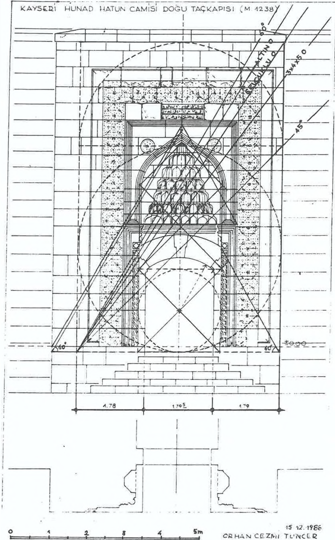
Çizim 19: Modülasyon denemeleri.
