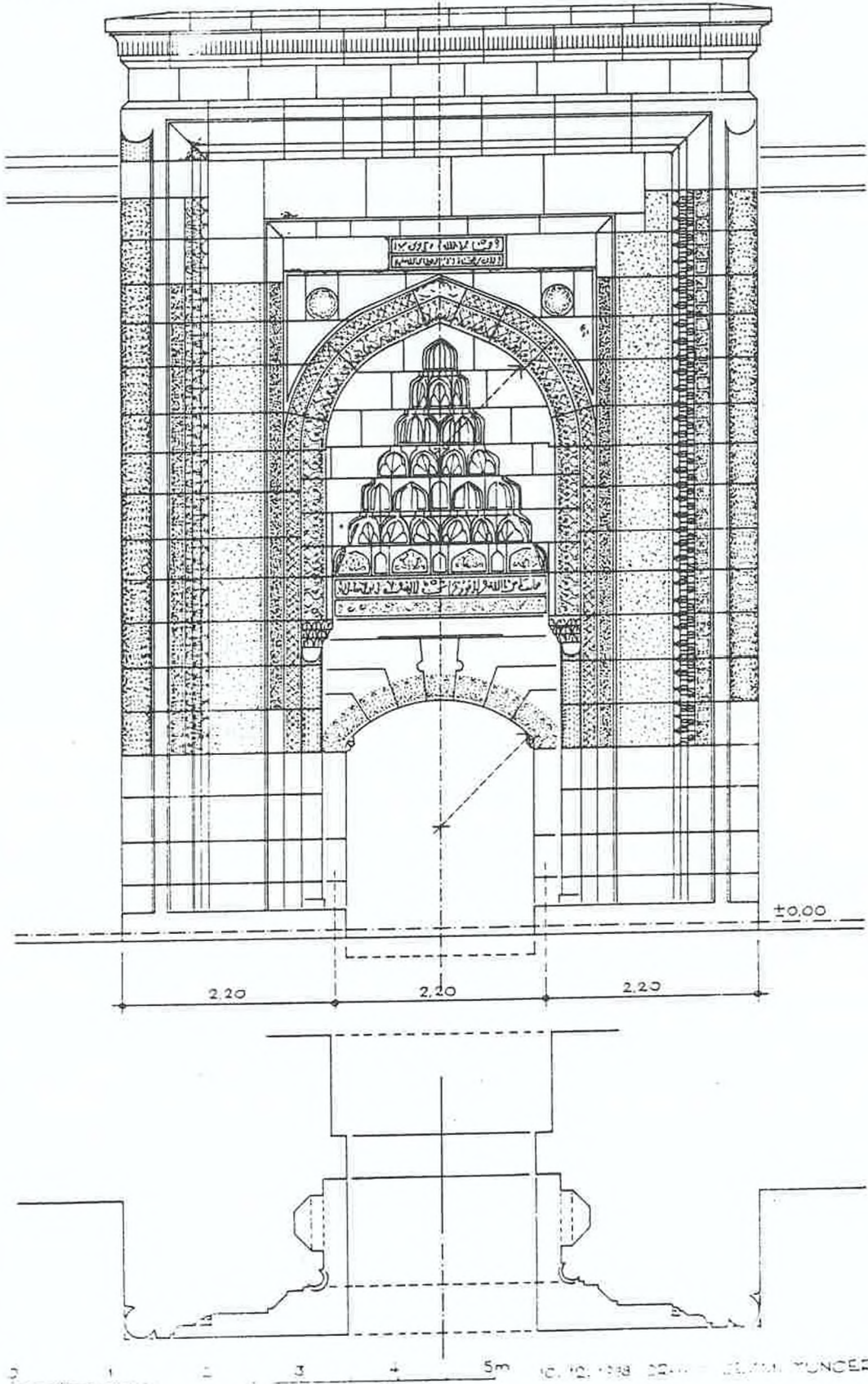
Çizim 23: Hacı Kılıç Medresesi taçkapısı rölövesi.
