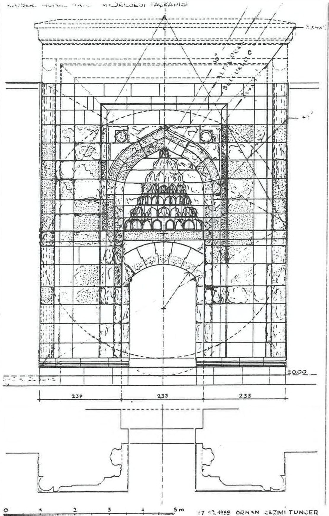
Çizim 12: Modülasyon denemeleri.
