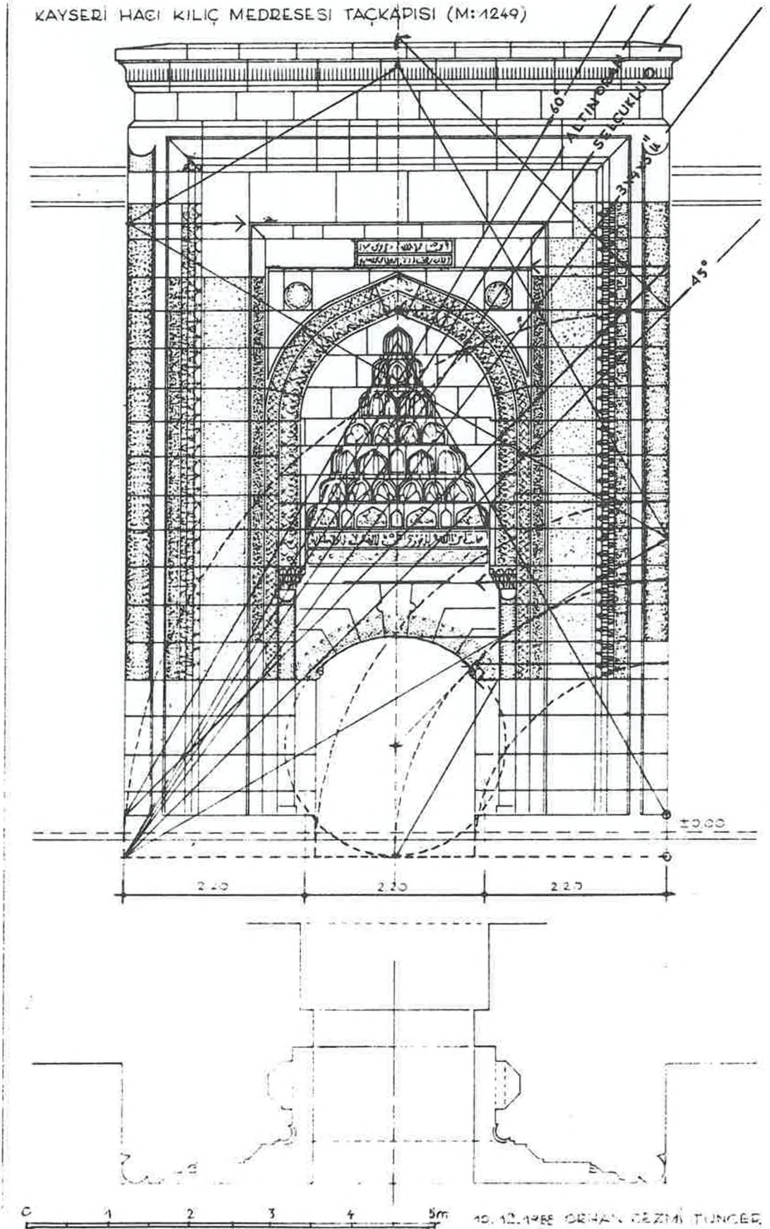
Çizim 26: Modülasyon denemeleri.
