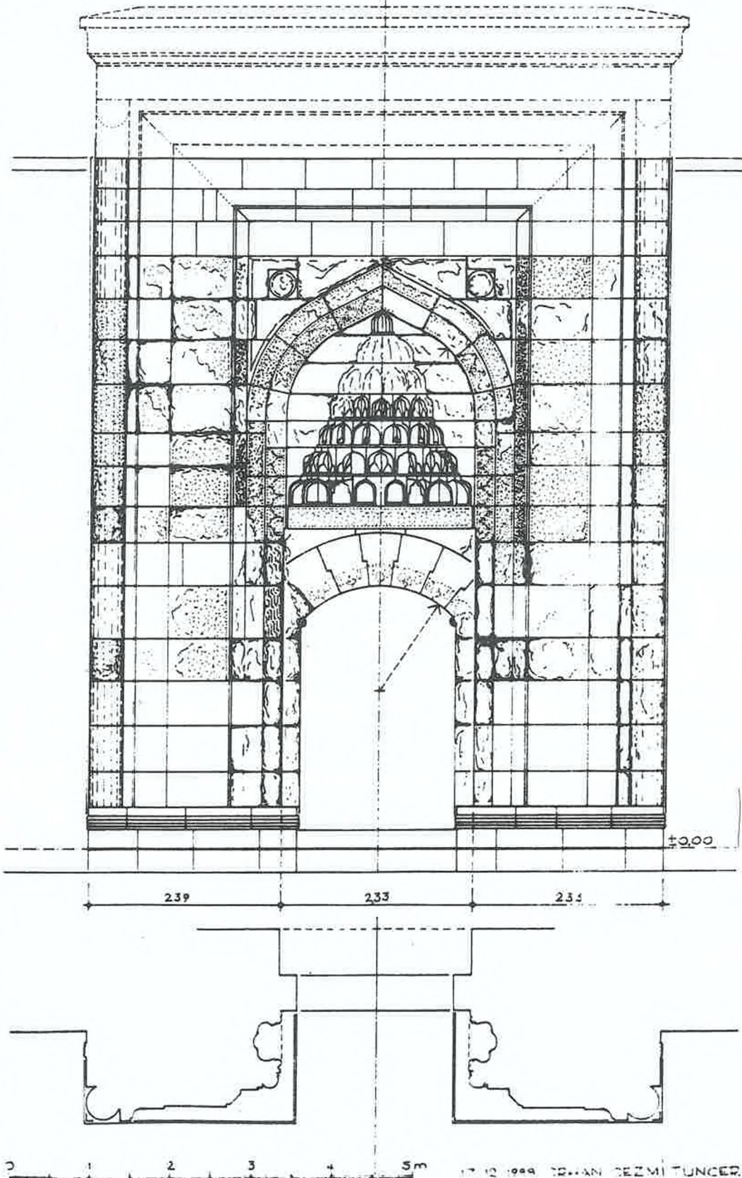
Çizim 9: Hunat Hatun Medresesi taçkapisı rölövesi.
