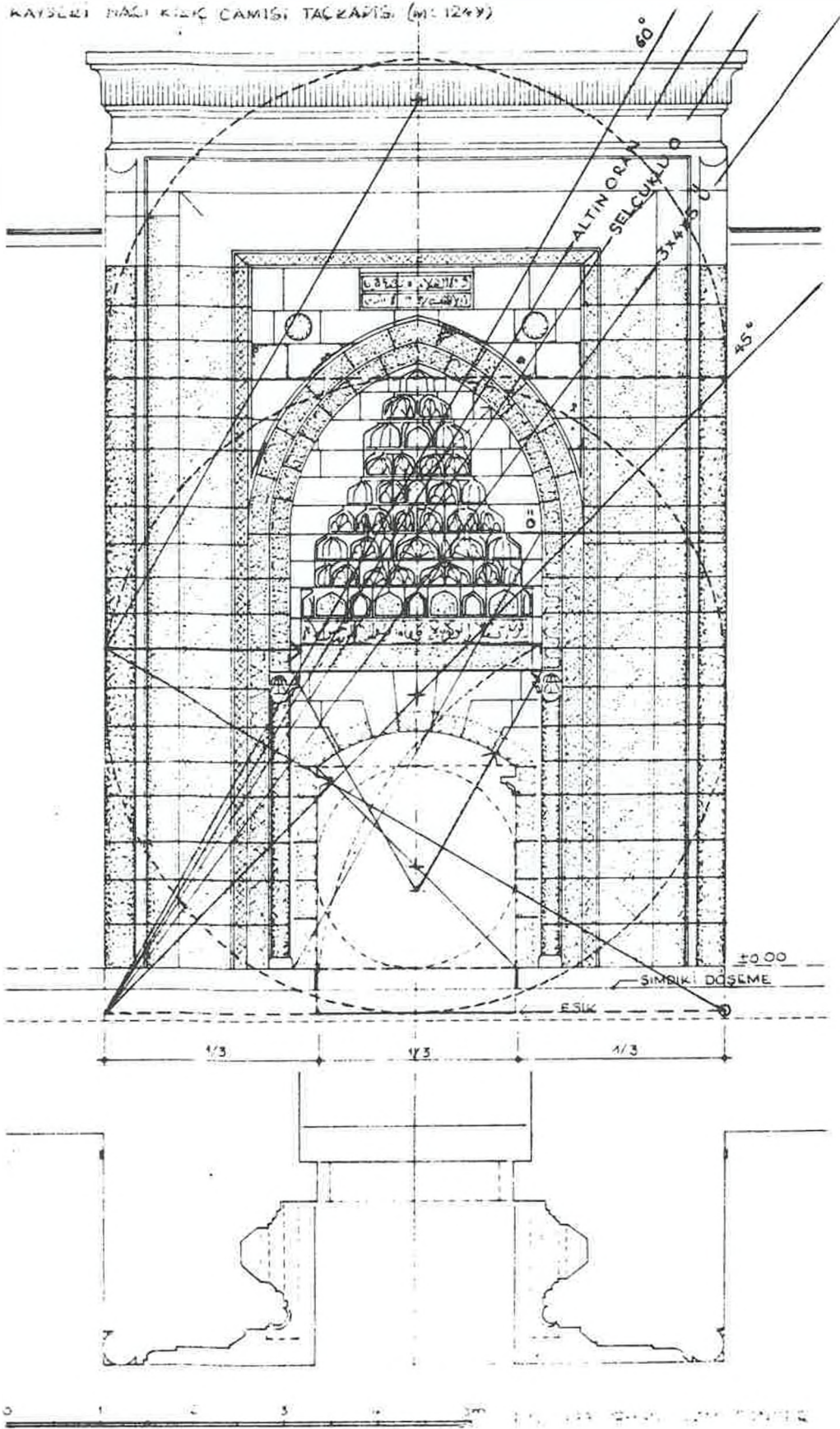
Çizim 22: Modülasyon denemeleri.
