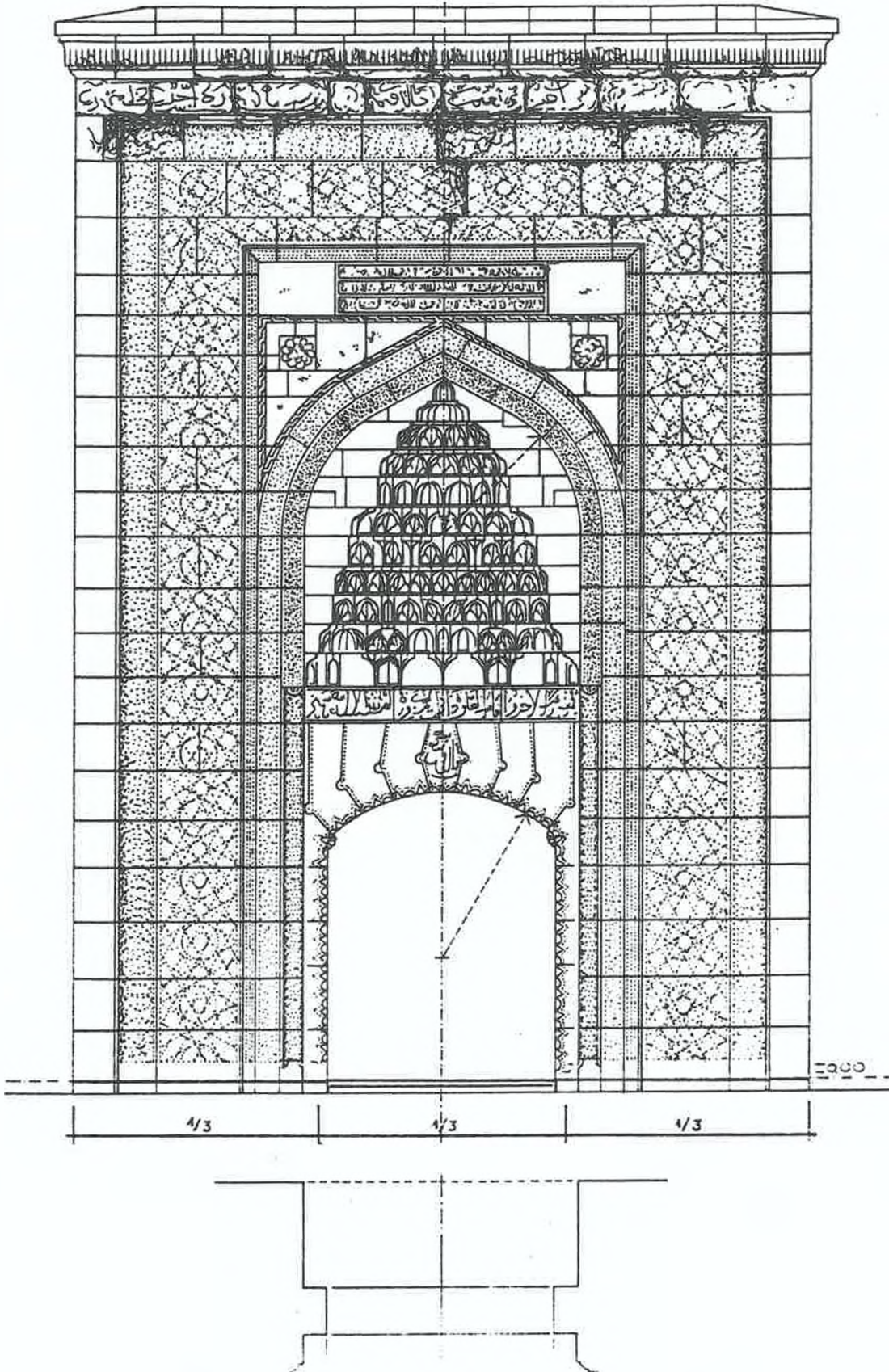
Çizim 13: Hunat Hatun Camisi batı taçkapısı rölövesi.
