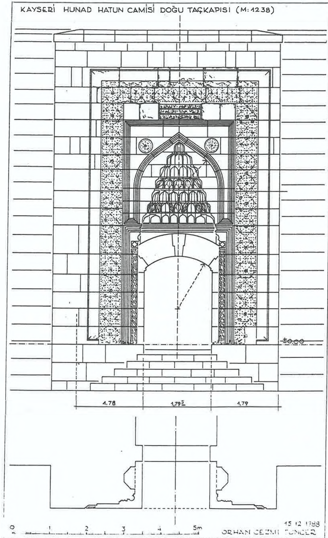
Çizim 17: Hunat Hatun Camisi doğu taçkapısı rölövesi.
