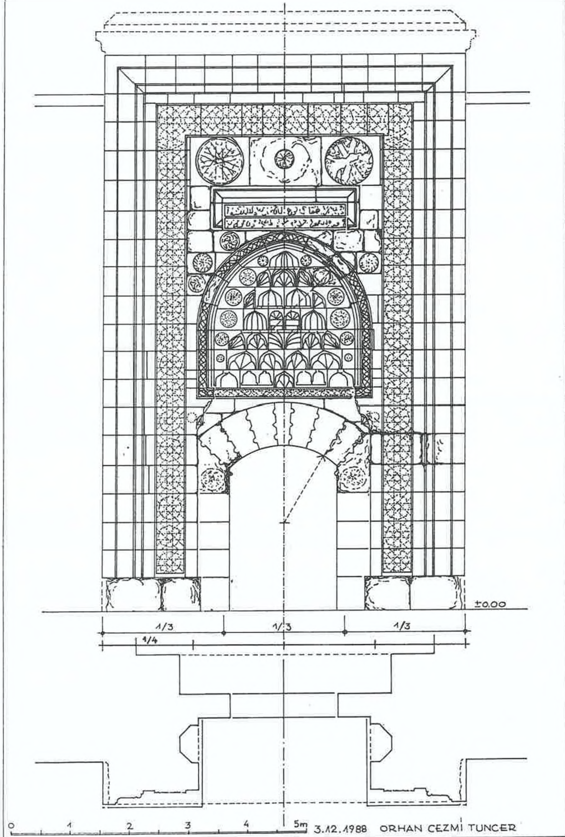
Çizim 1: Geyher Nesibe Şifahanesi taçkapisı rölövesi.
