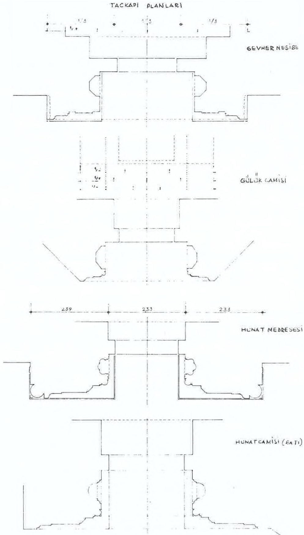
Çizim 27: Taçkapı planları.
