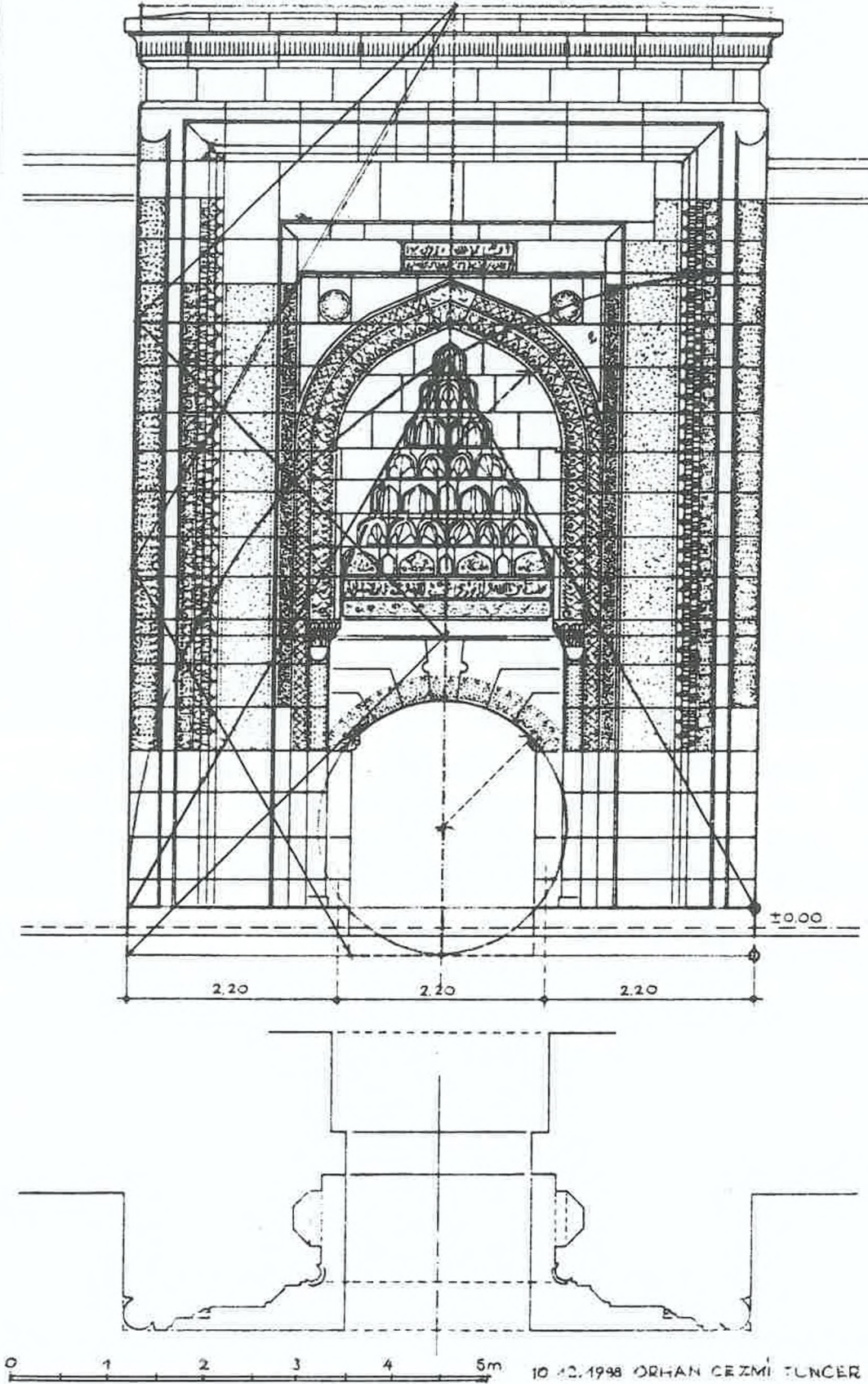
KAYSERİ HACI KILIÇ MEDRESESİ TAÇKAPISI (M:1249)
