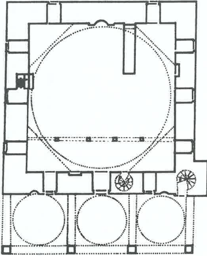
Plan:6 Camli
