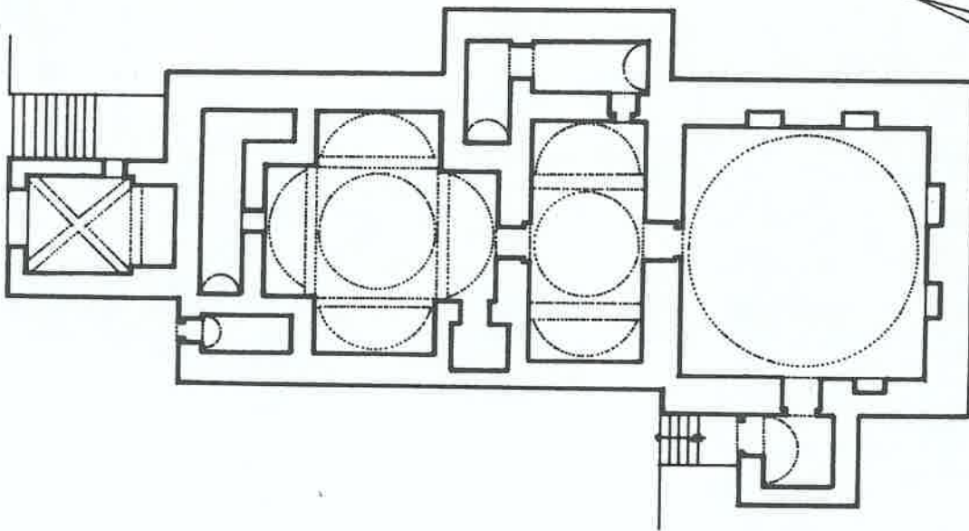
Plan:10. Hamam
