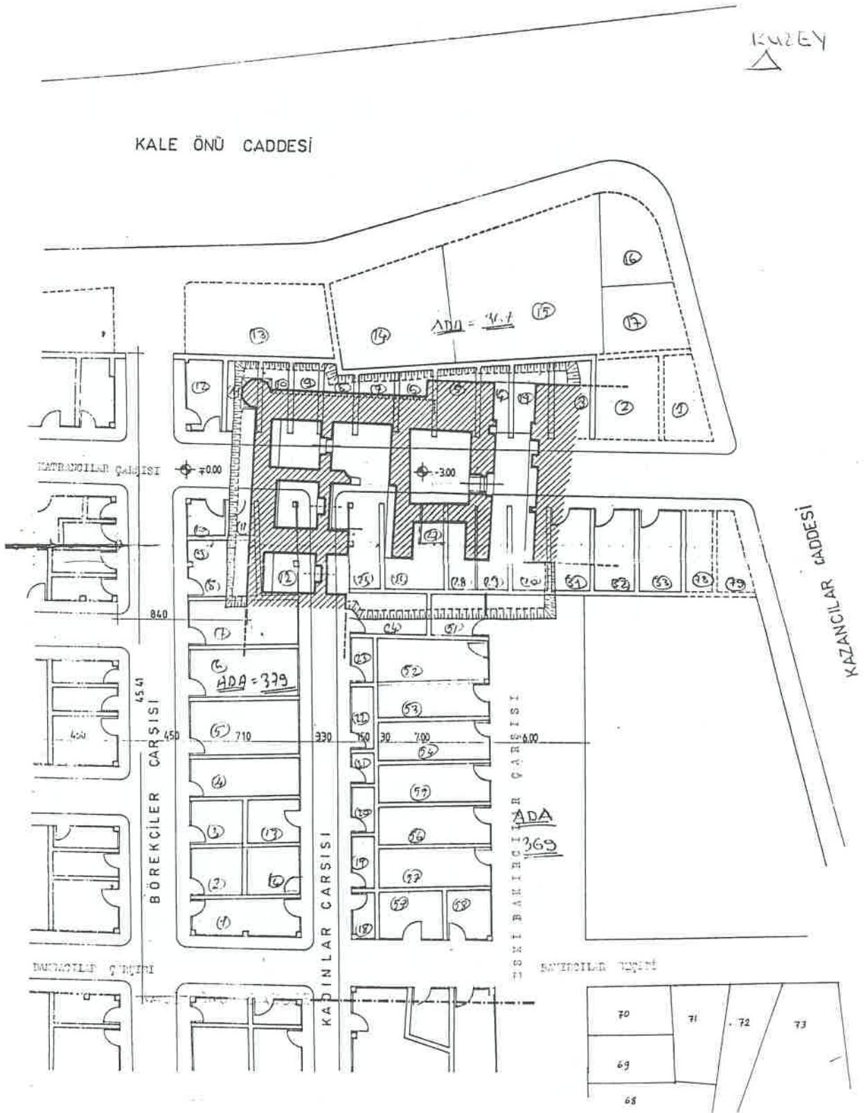
PLAN- PERVANEBEY MEDRESESİNİN KAPALI ÇARŞIDAKİ YERİ
