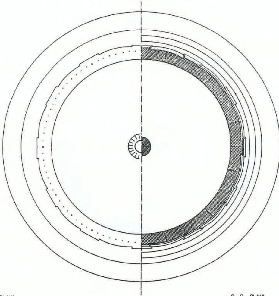
A-A PLANI
