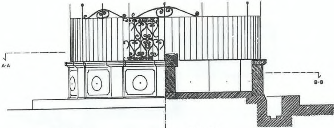
KİSMİ CEPHE
