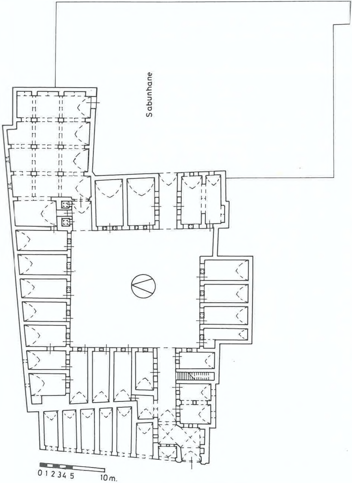
Çizim 7: Gaziantep Kürkcü Hanı, alt kat planı.
