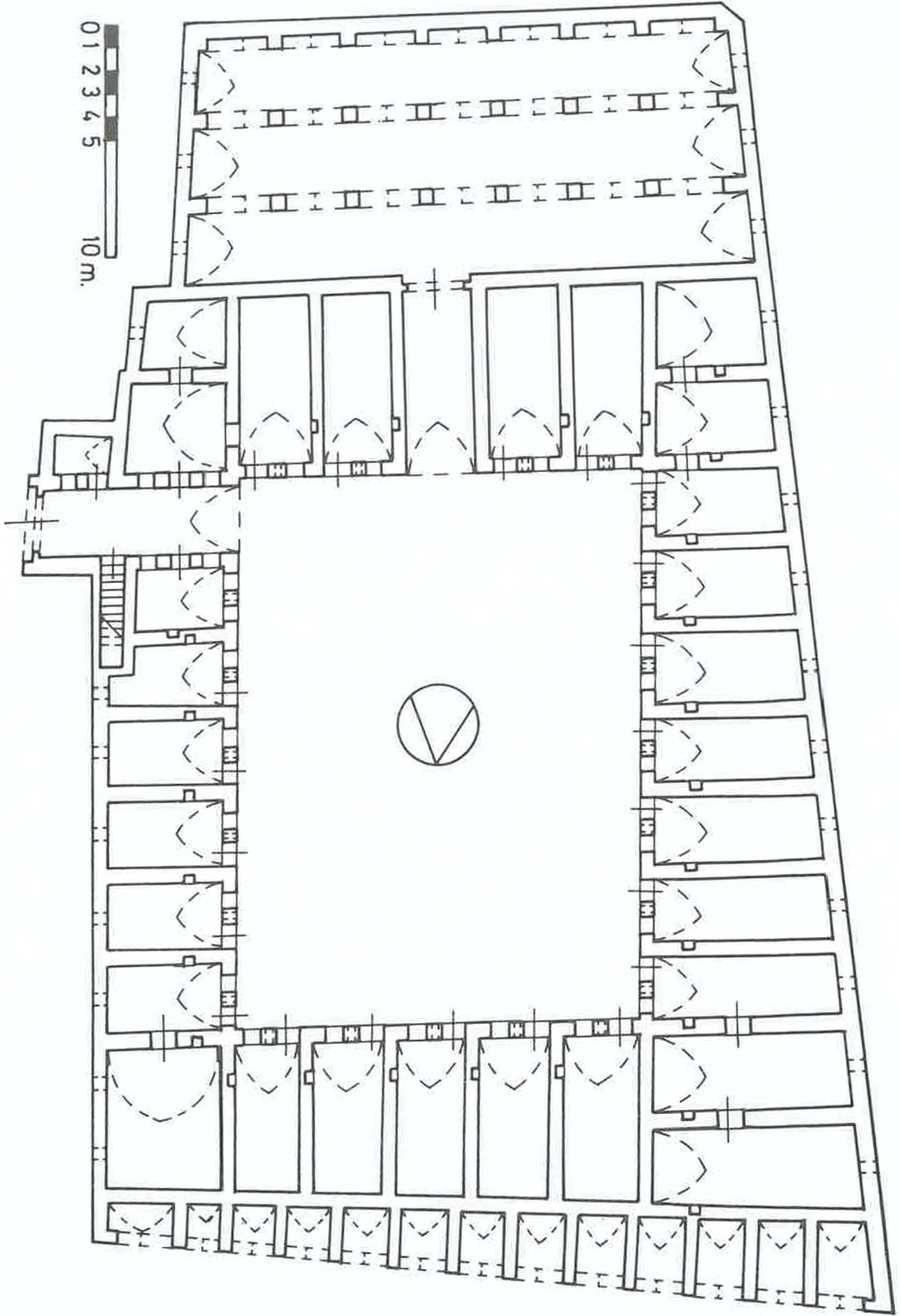
Çizim 3: Gaziantep Millet Hanı, alt kat restitüsyon planı (Gaziantep Belediyesi'nden işlenerek).
