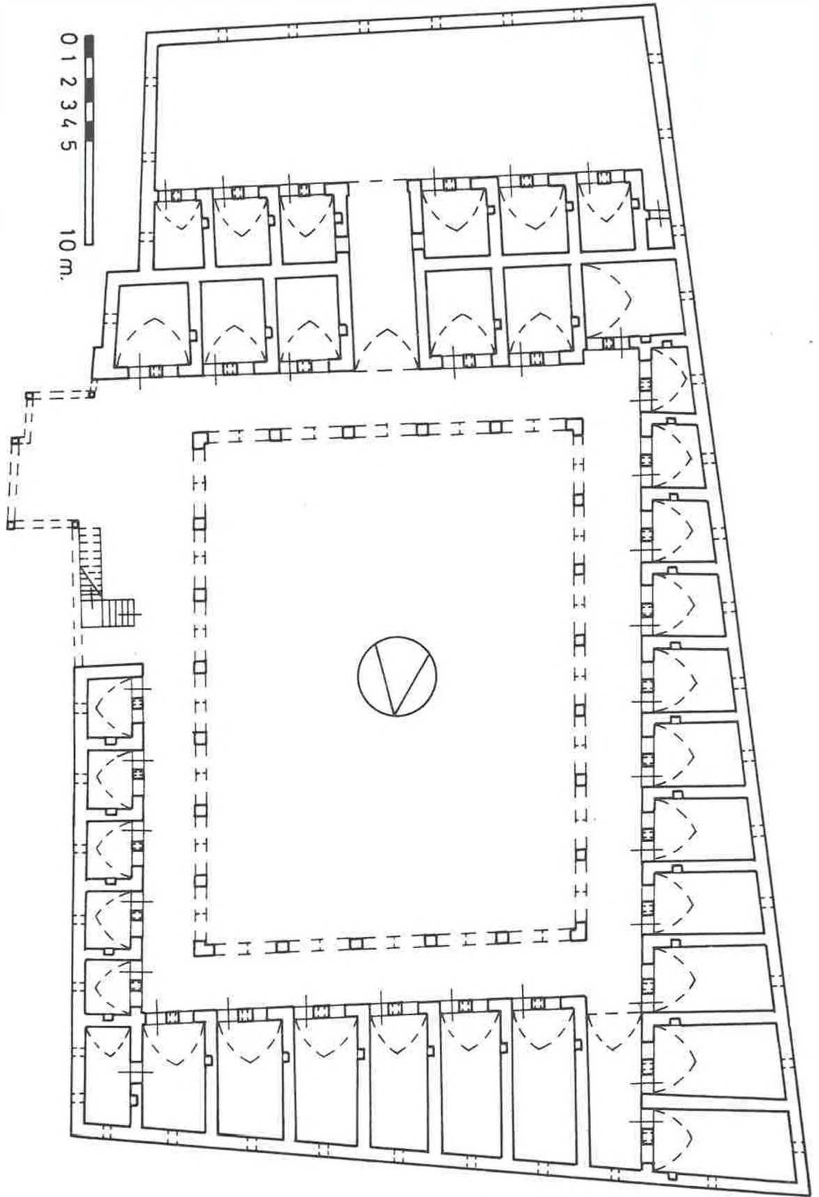
Çizim 4: Gaziantep Millet hanı, üst kat restitüsyon planı (Gaziantep Belediyesi'nden işlenerek).
