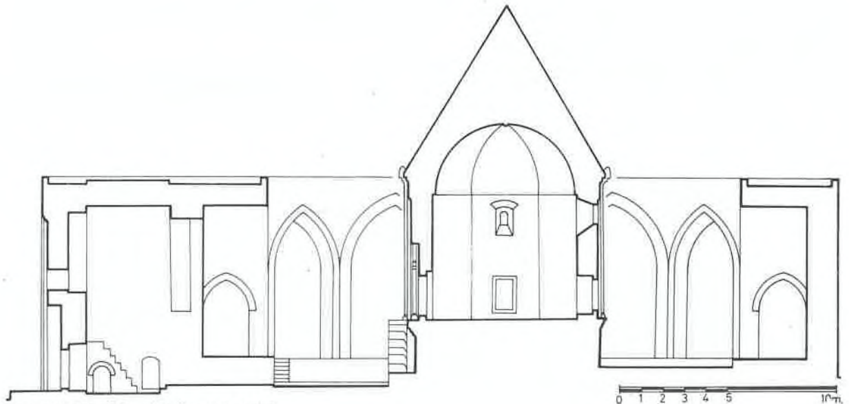
Şekil 4. KAYSERİ, KÖSK HÂNIKÂHI, B-B KESİTİ (Vakıflar Genel Müdürlüğü Arşivi'nden düzeltilerek)
