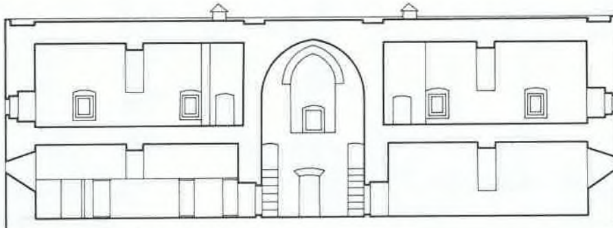
Sek.3. KAYSERİ, KÖŞK HÂNIKÂHI, A-A KESİTİ (Vakıflar Genel Müdürlüğü Arşivinden düzeltilerek)
