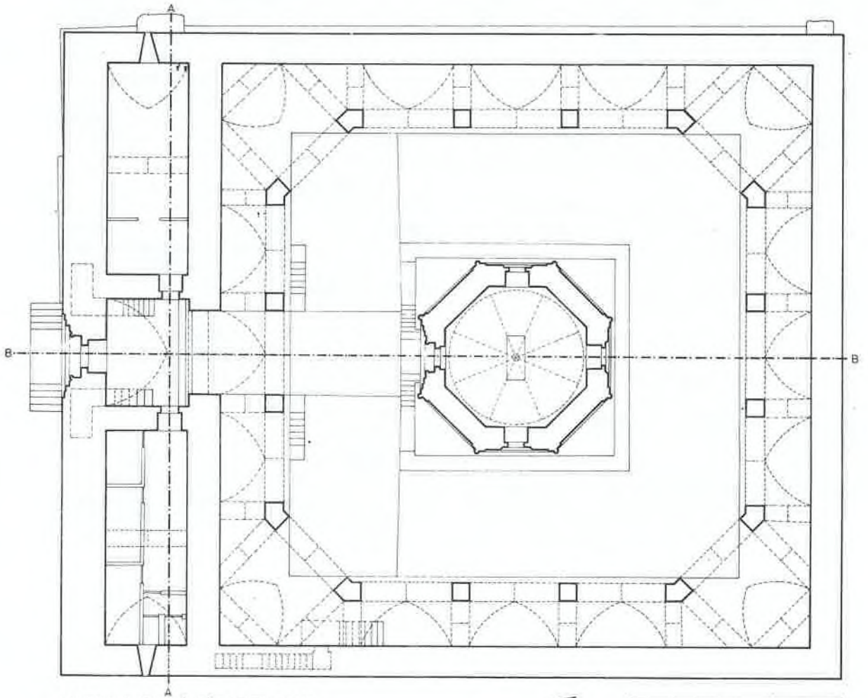
Şekil 1. KAYSERİ, KÖSK HÂNIKÂHI, ROLOVE PLANI (Vakıflar Genel Müdürlüğü Arşivi'nden düzeltilerek)
