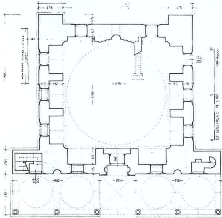
İstanbul Bâli Paşa Câmii'nin planı (İ. Aydın Yüksel'den alınmıştır).
