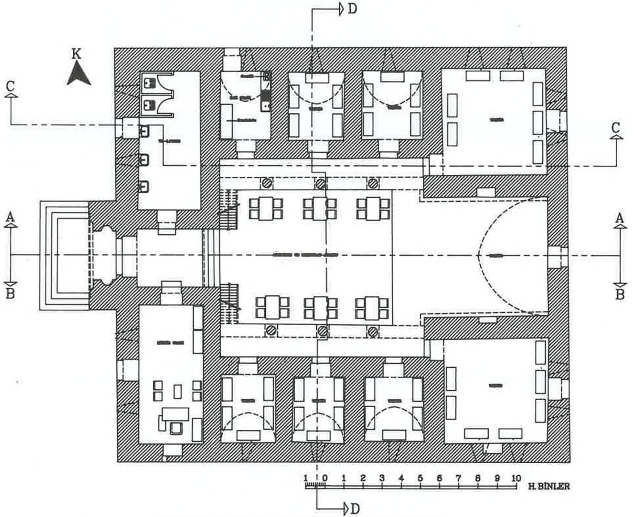
ŞEKİL 17, ALT KAT PLANI KULLANIM
