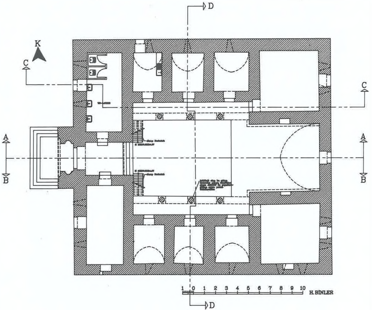
ŞEKİL: 9, ALT KAT PLANI RESTORASYON
