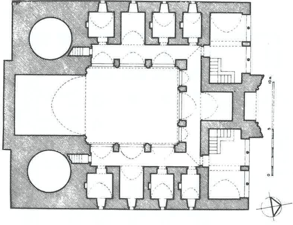
Şekil 22: Niğde Ak Medrese üst kat planı (A. Kuran)
