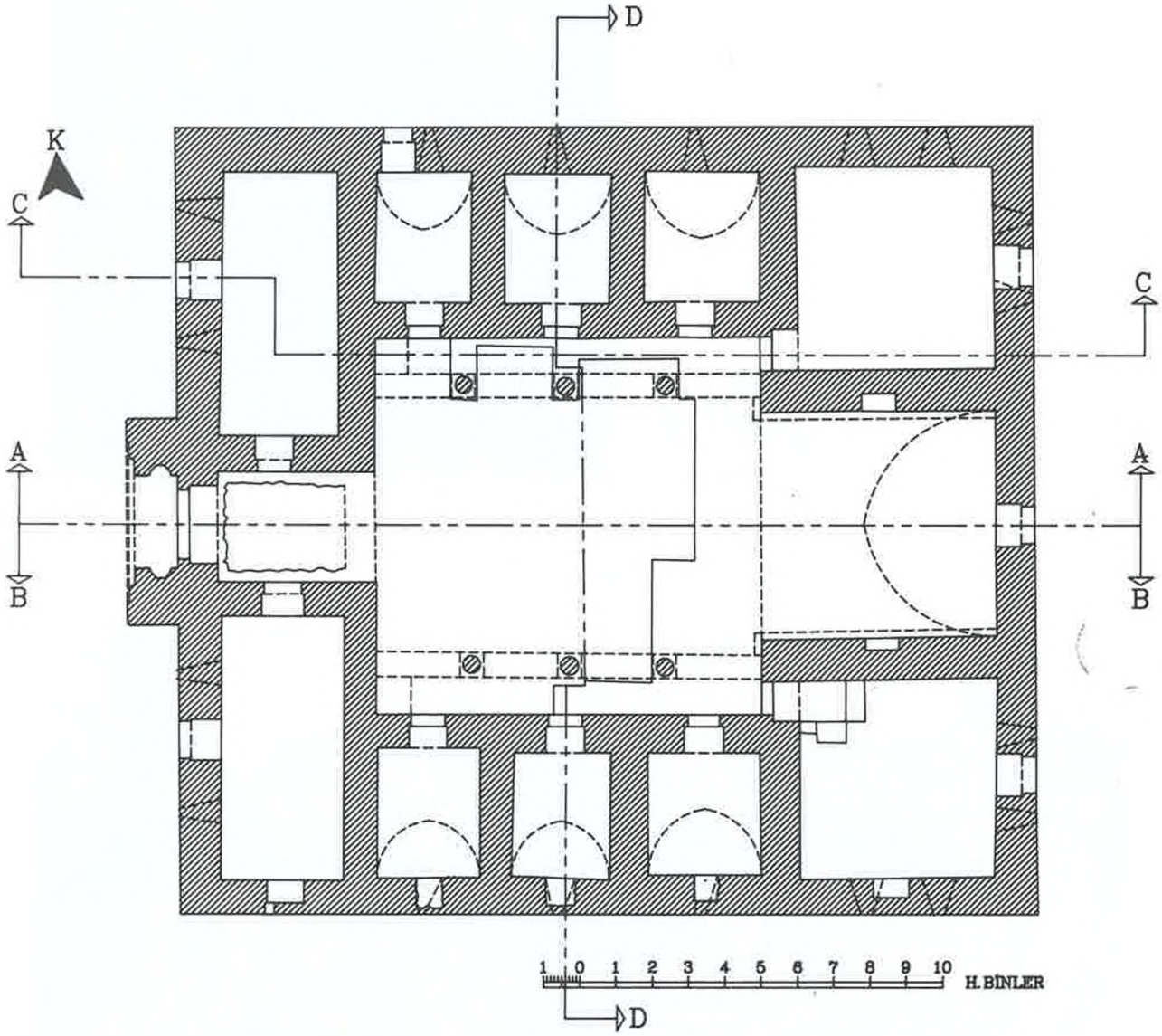
ŞEKİL: 1, ALT KAT PLANI RÖLÖVE
