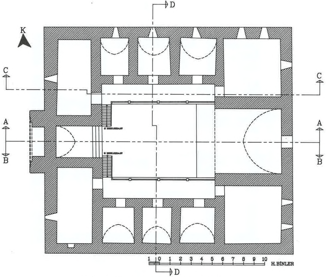
ŞEKİL 10, ÜST KAT PLANI RESTORASYON
