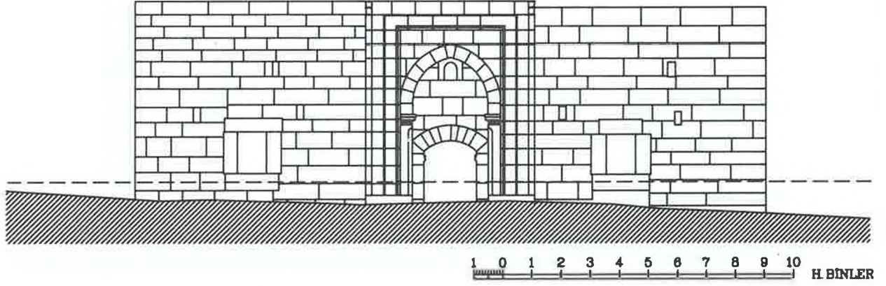
ŞEKİL 7, ÖN CEPHE RÖLÖVE
