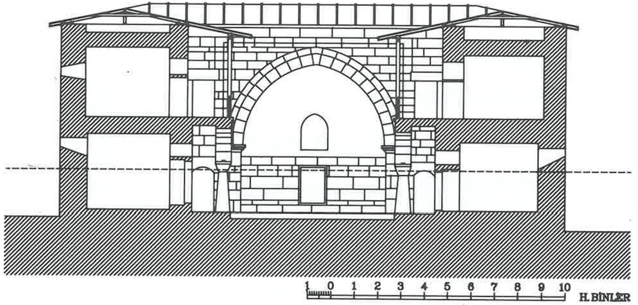
ŞEKİL: 14, D-D KESİTİ RESTORASYON
