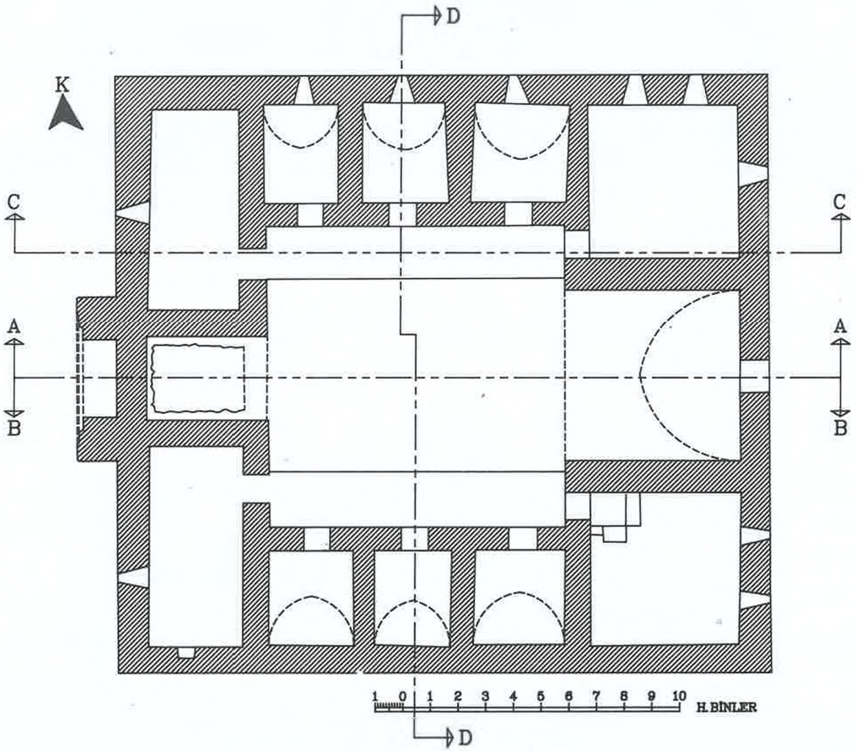
ŞEKİL: 2, ÜST KAT PLANI RÖLÖVE
