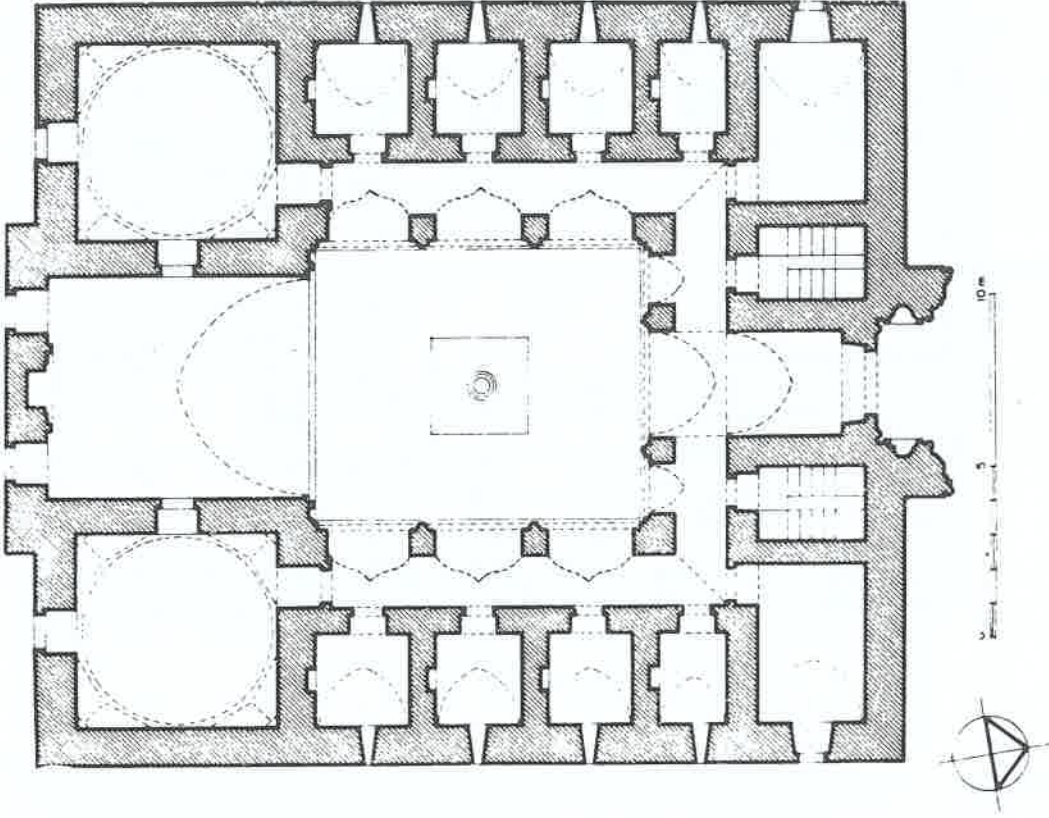
Şekil 21: Nigde Ak Medrese alt kat planı (A. Kuran)
