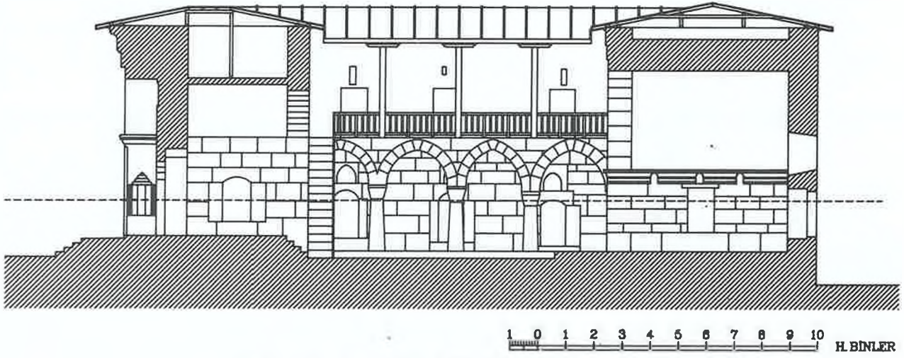
ŞEKİL 11, A-A KESİTİ RESTORASYON
