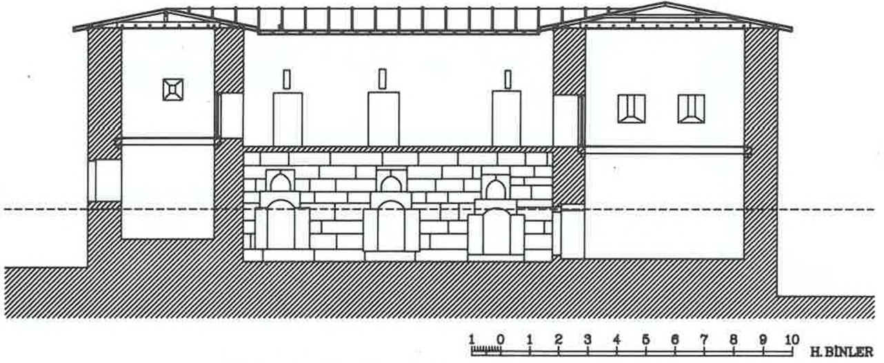
ŞEKİL: 13, C-C KESİTİ RESTORASYON
