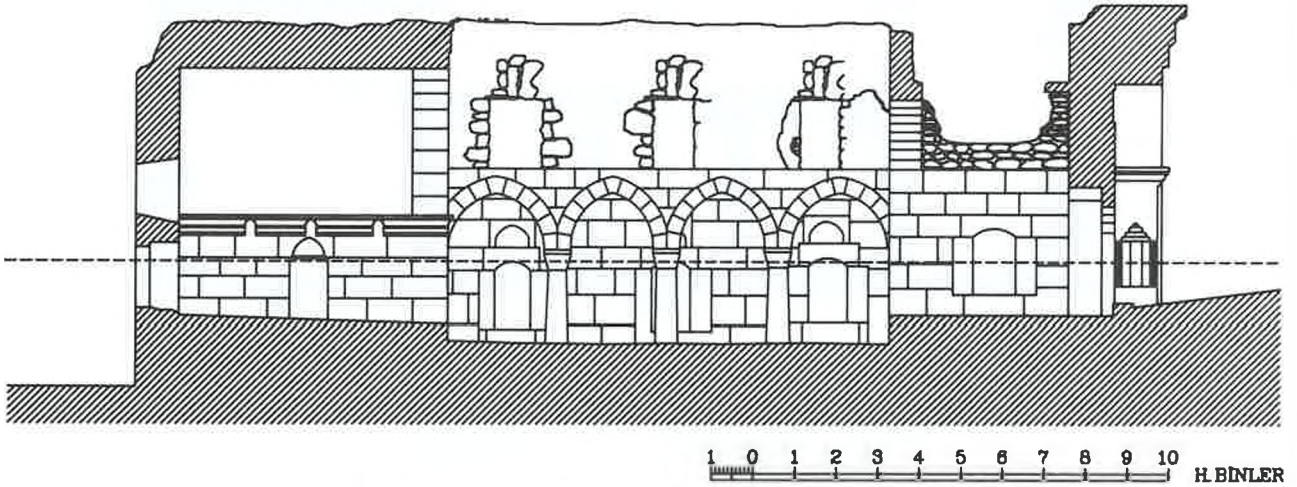
ŞEKİL: 4, B-B KESİTİ RÖLÖVE
