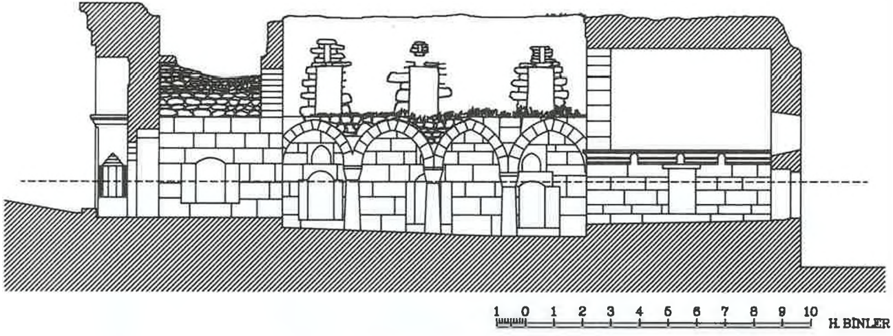
ŞEKİL: 3, A-A KESİTİ RÖLÖVE
