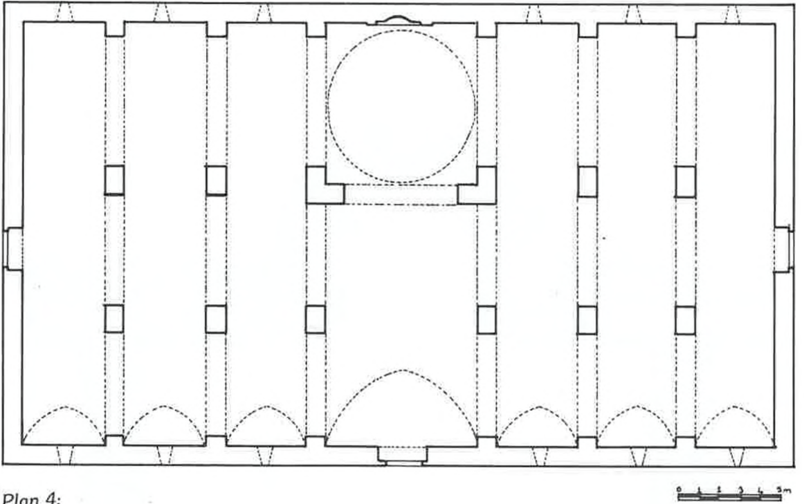
KONYA İPLİKÇİ CAMİ RESTİTÜSYON PLANI (H. Karamağaralı'dan)
