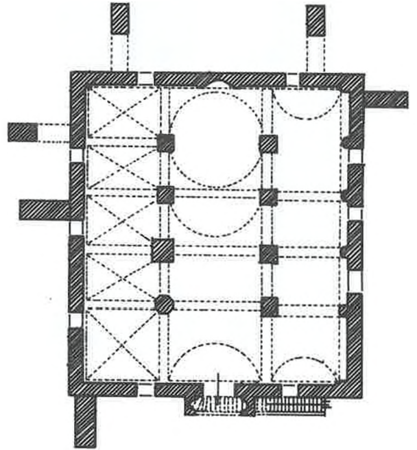
KONYA İPLİKÇİ CAMİ RESTİTÜSYON PLANI (H. Karamağaralı'dan)
