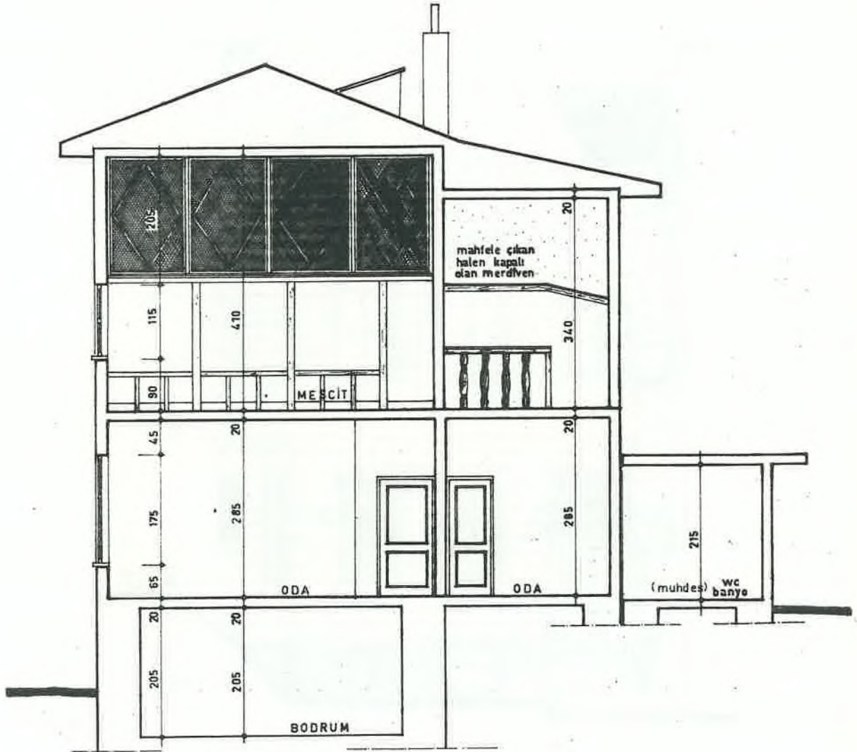
A-A KESİTİ 1/50
