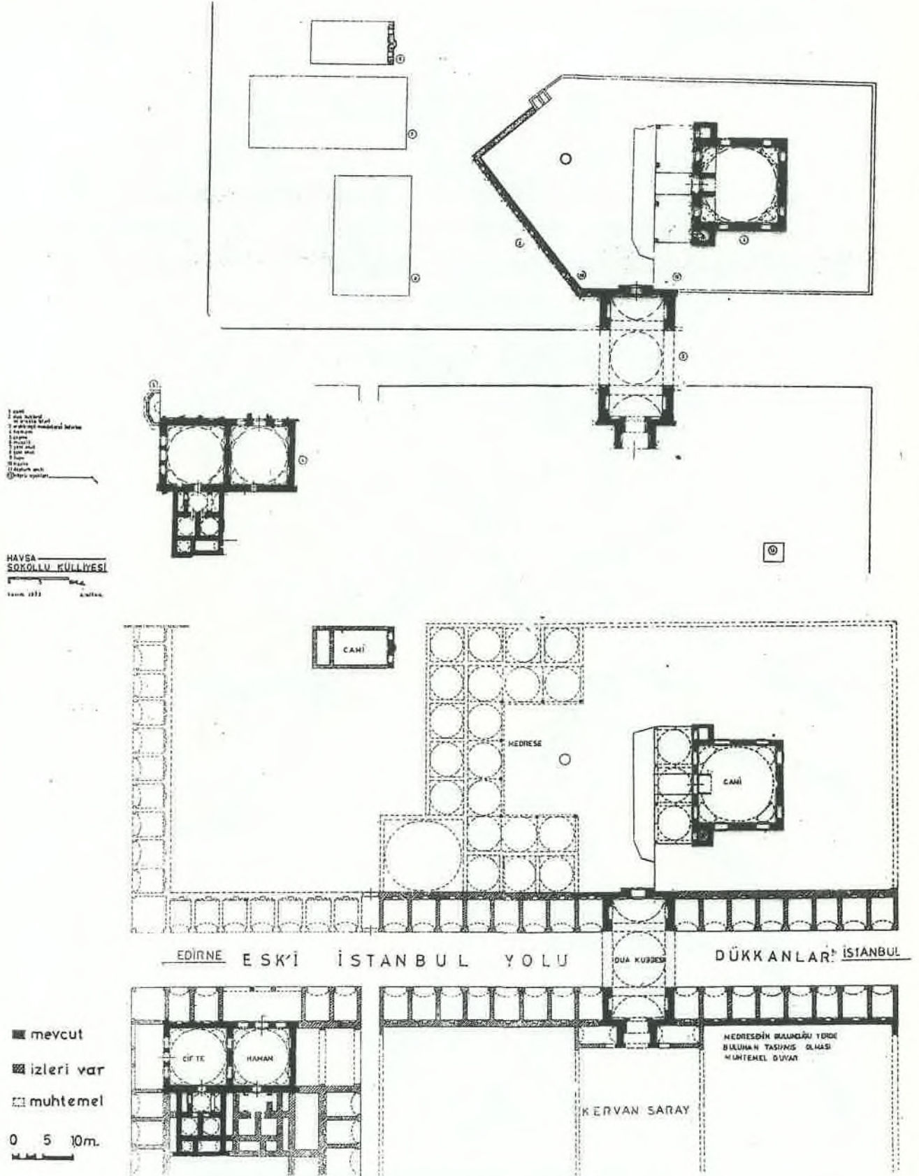
Şekil No 8: Havsa, Mimar Sinan yapıları ile ilgili bir Restitüsyon Çalışması (1988) (Bkz. Tablo Menzil No.7)
