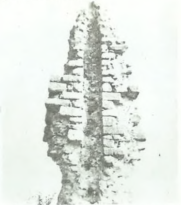
Foto No 9: Lüleburgaz/Büyükkarıştıran 3'nolu Su terazi kulesi (Bkz Tablo, Menzil No:4)
