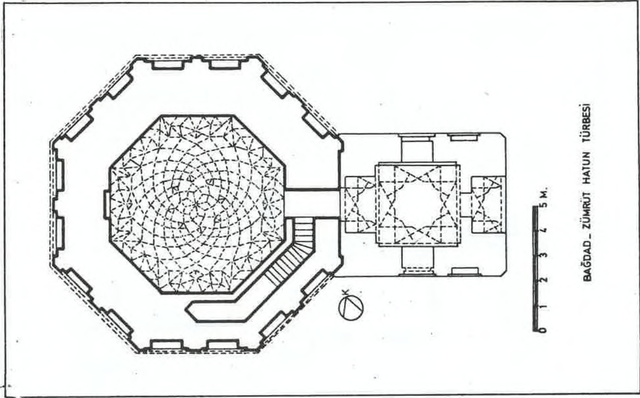
Çizim 2: Bağdad-Zümrüt Hatun Türbesi
