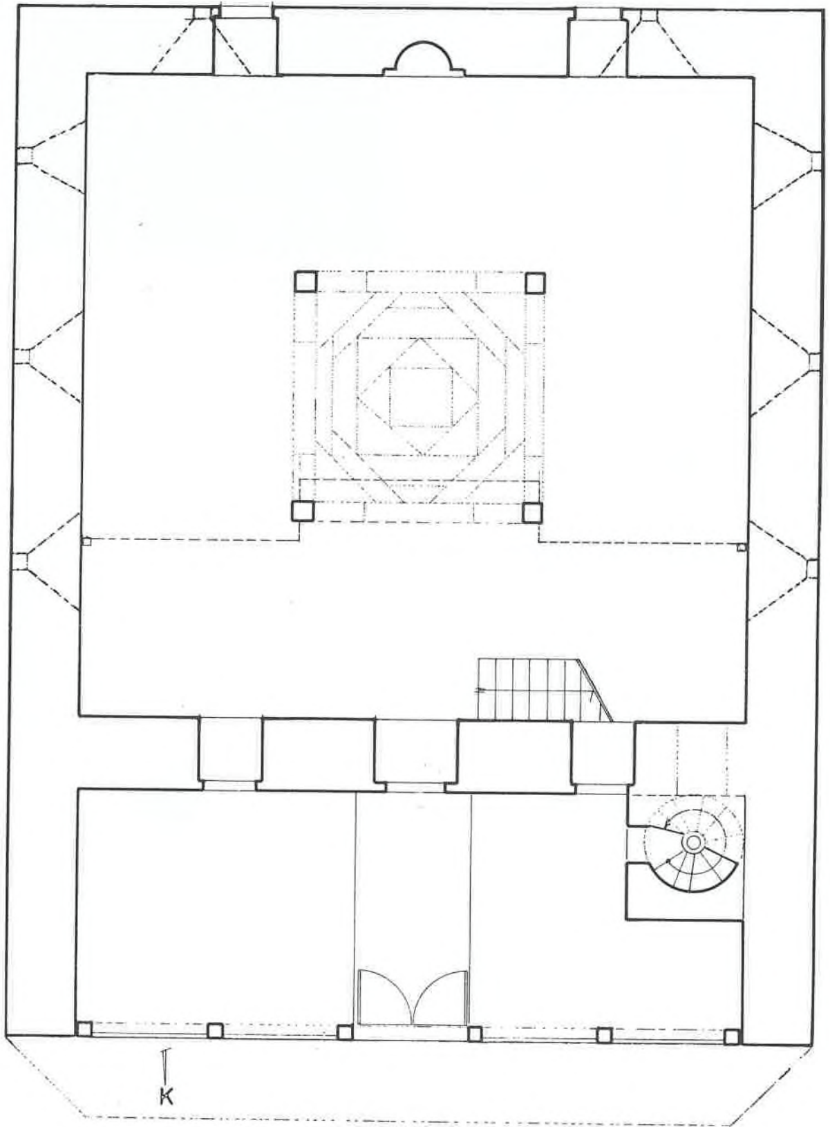
ŞEKİL - 3 : Kümbet Köyü Hacı Osman Efendi Camii planı.
