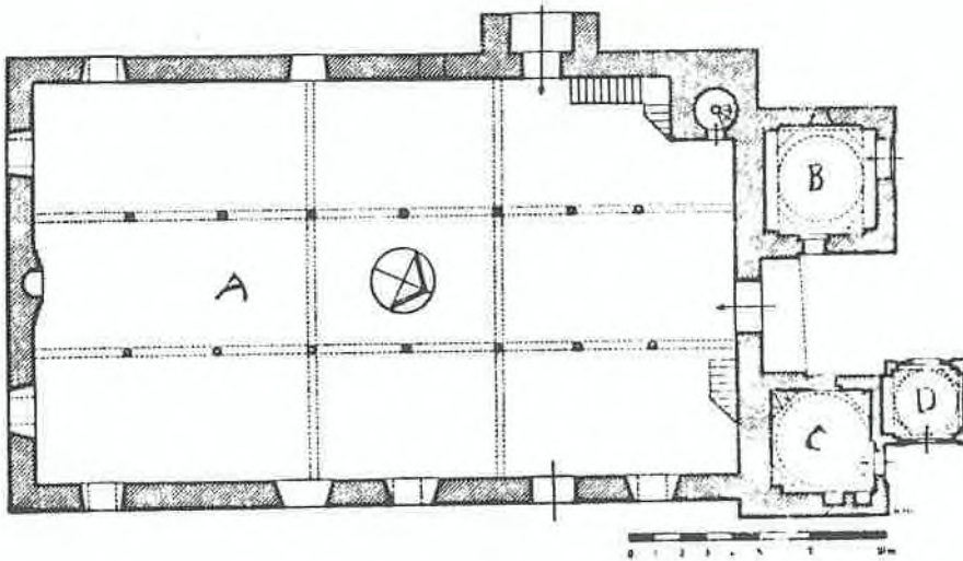
Plân - 1 : Seyyid Harun Camii ve bitişindeki Türbeler Plânı. A- Cami, B- Seyyid Harun Türbesi, C- Halife Sultan Türbesi, D- Rüstem Bay Türbesi (R. Hüseyin ÜNAL'dan).
