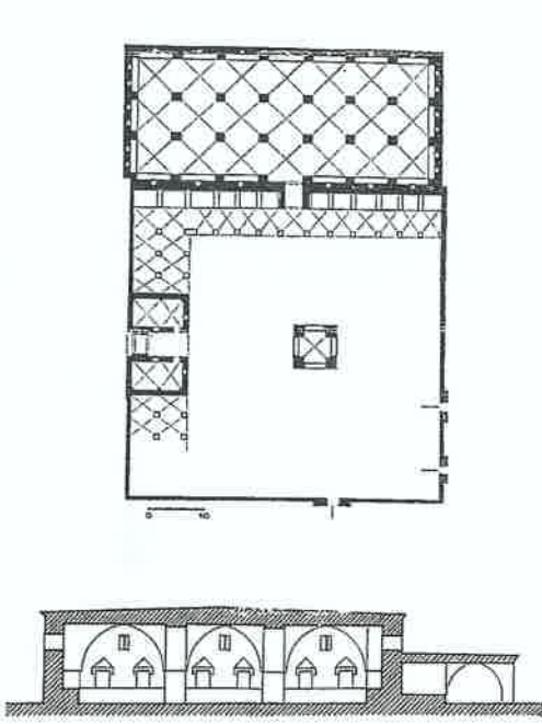
Lev. 37: DJISR ESH SHUGHUR Külliyesi, vaziyet planı (Sauvaget, 1937).
