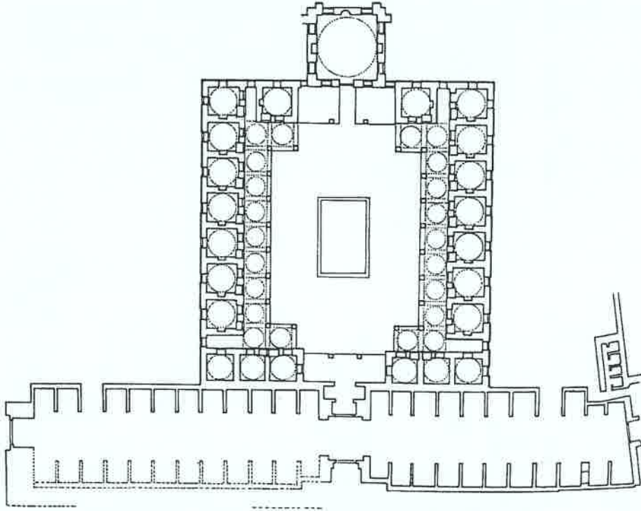
Lev. 23: ŞAM, Süleymaniye Külliyesi. Medrese Planı (Ahunbay, 1988).
