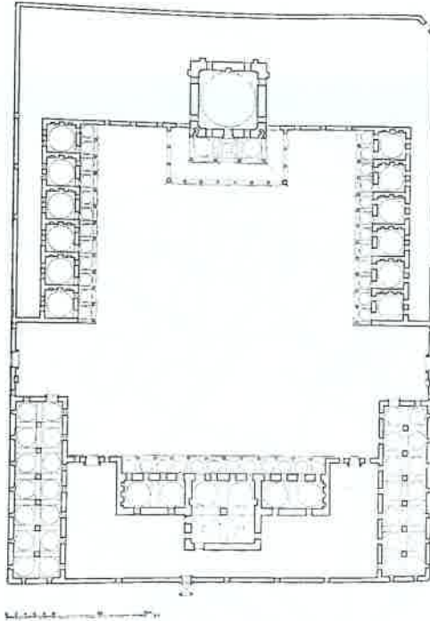
Lev. 8: ŞAM, Süleymaniye Külliyesi, Konum Planı (Kuran, 1986).
