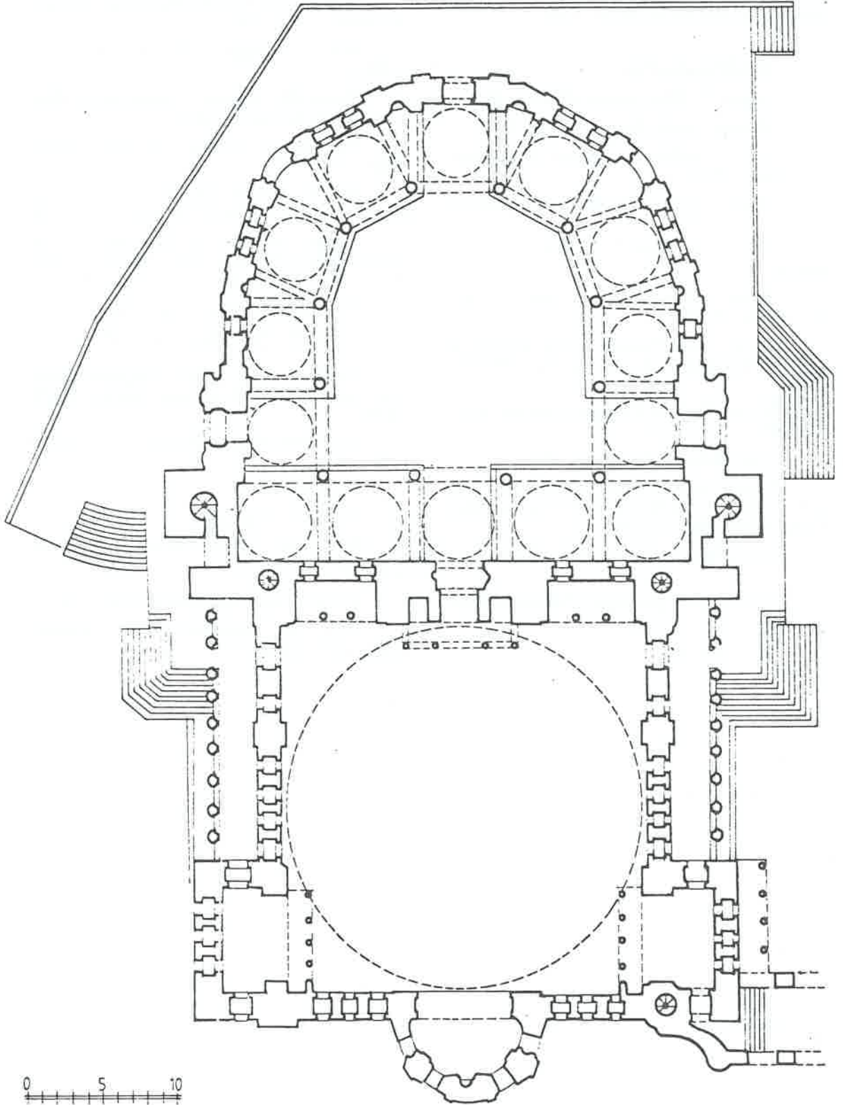
Nuruosmaniye Camii plânı (G. Goodwin'den)
