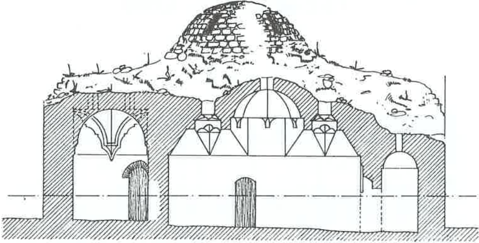
çizim: 10-a-a kesit
