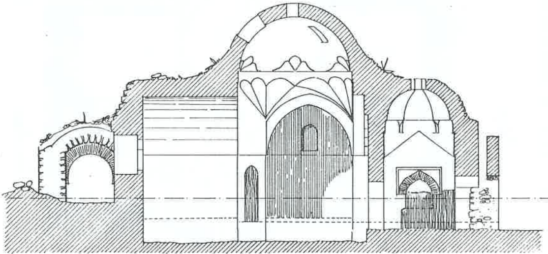
çizim: 11-b-b' kesit
