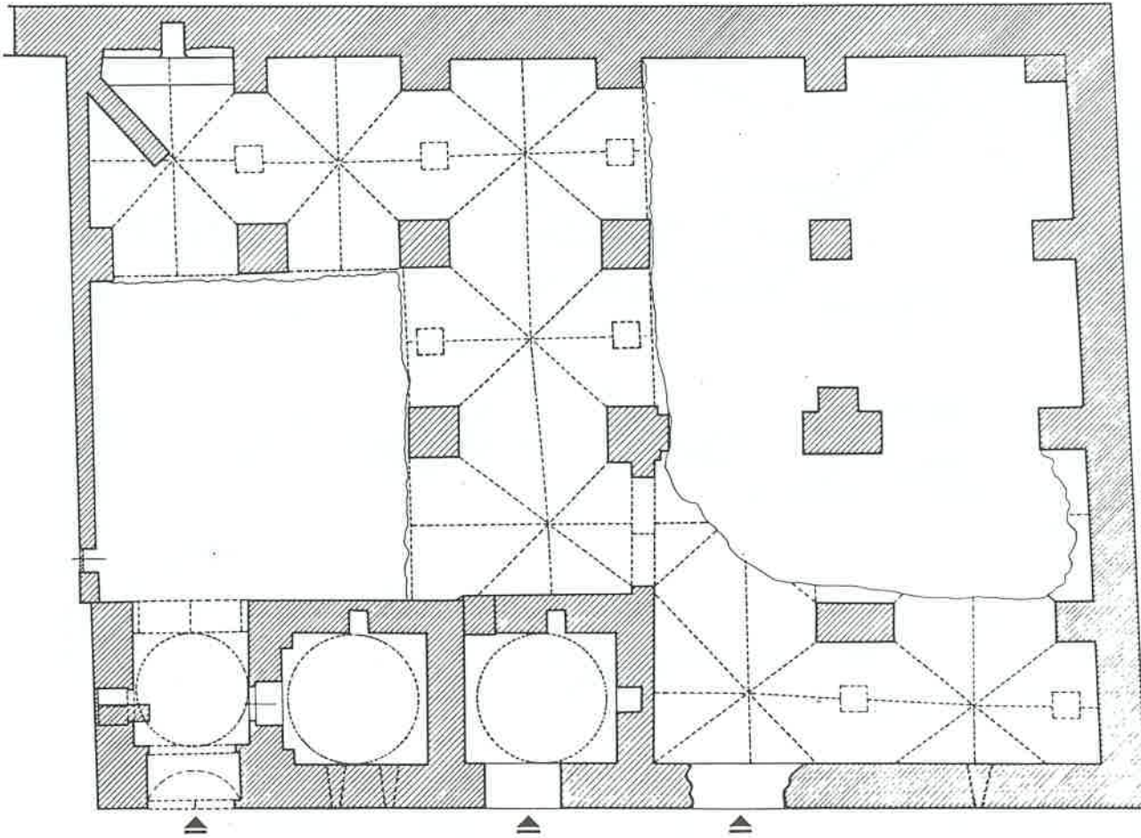
Lev. 18: Han, rölöve planı (1990, F. Ertuğ).
