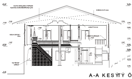
Kesit A-A
