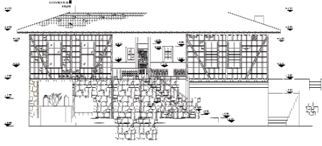
Güney Cephesi
