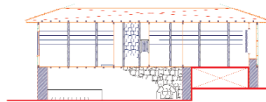
Kesit A-A
