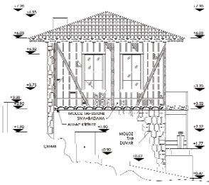
Batı Cephesi
