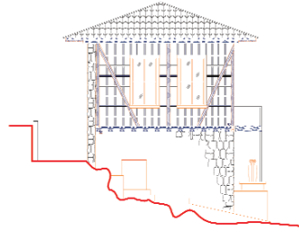
Batı Cephesi
