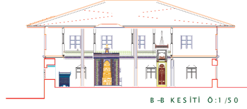
B-B KESİTİ Ö:1/50
