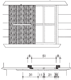
PENCERE İÇ GÖRÜŞÜ
