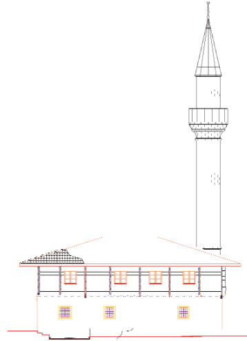
Güney Cephesi
