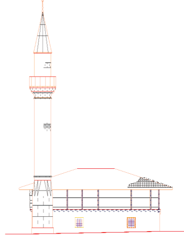
Kuzey Cephesi
