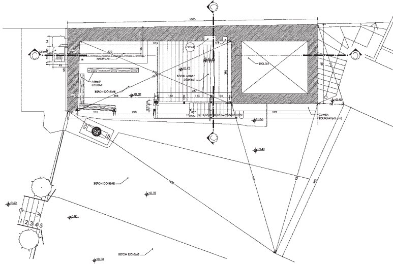
ZEMİN KAT PLANI Ö: 1/50
