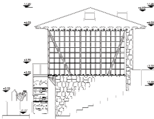
Doğu cephesi
