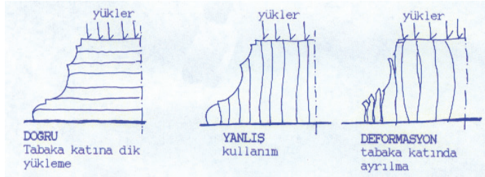
Şekil 5. Ocaktaki tabakalanma yönüne göre doğru/yanlış kullanım biçimi (Küçükkaya, 2003)
