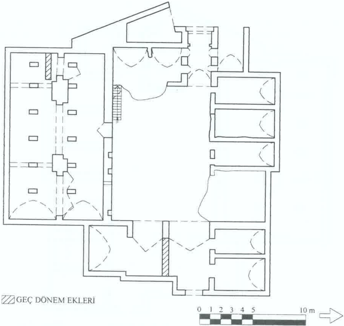
Çizim 18: Şaban Hanı zemin kat rölöve planı (Rölöve: A. Özme-L. Özbek).
