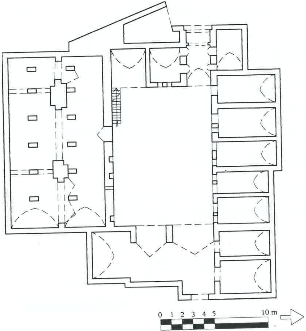
Çizim 19: Şaban Hanı zemin kat restitüsyon planı.
