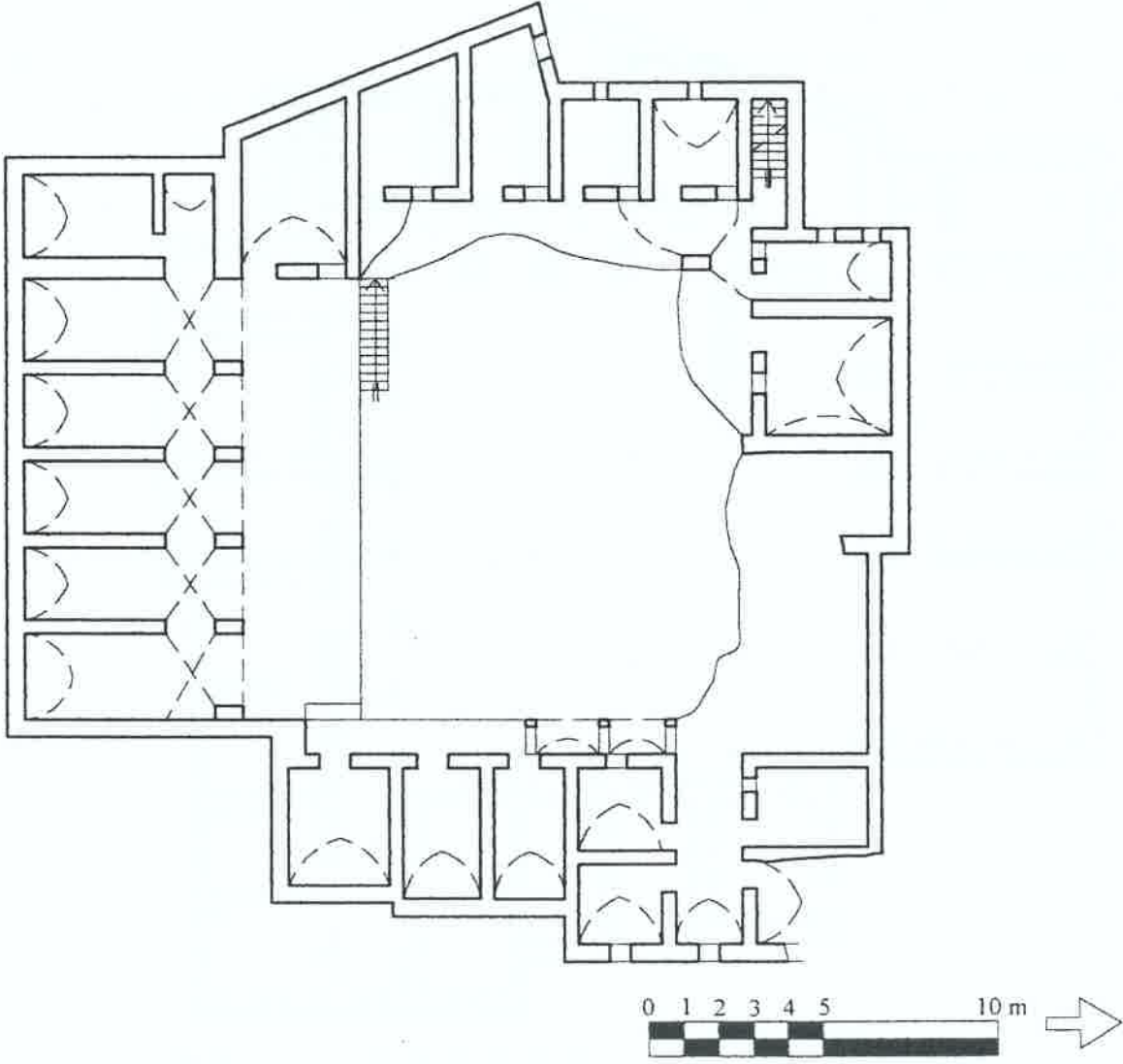
Çizim 20: Şaban Hanı birinci kat rölöve planı (Rölöve: A. Özme-L. Özbek).
