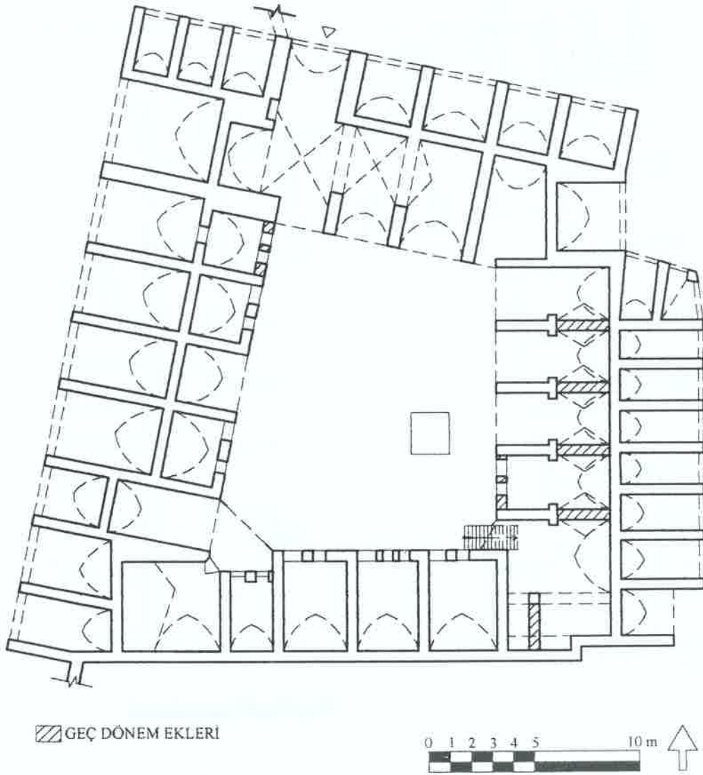
Çizim 22: Mençek Hanı zemin kat rölöve planı (Rölöve: A. Özme-L. Özbek).
