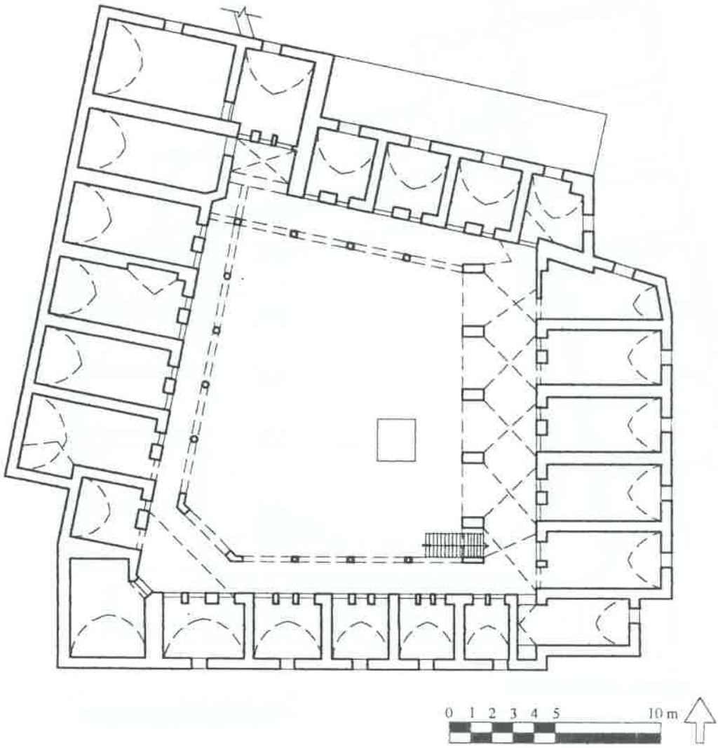
Çizim 25: Mençek Hanı birinci kat restitüsyon planı.
