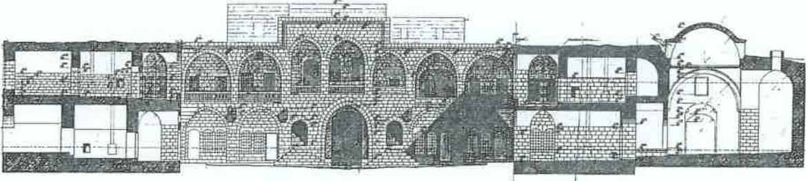
Çizim 13: Gümrük Hanı kuzey-güney kesiti (O. Cezmi Tuncer'den).
