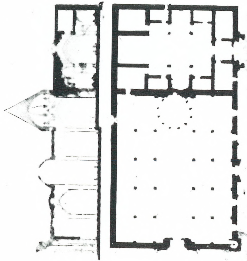
6 — Divriği'de Darüşşifa ve Ahmet Paşa camii'nin plân ve makta'ları ve darüşşifanın esas kapısı (A. Gabriel)
