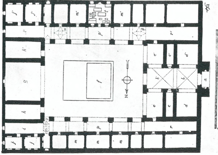
8 — Sivas Darüşşifası plânı (A. Gabriel)
