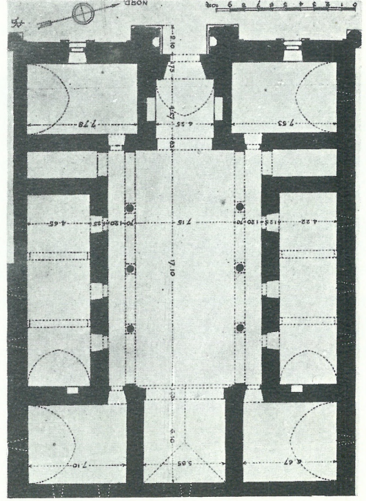
4 — Amasya Darüşşifası plânı (A. Gabriel)
