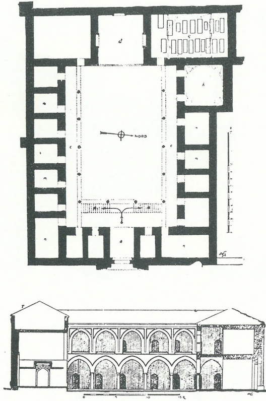
10 — Tokat Darüşşifası zemin kat plânı ve maktâı.
