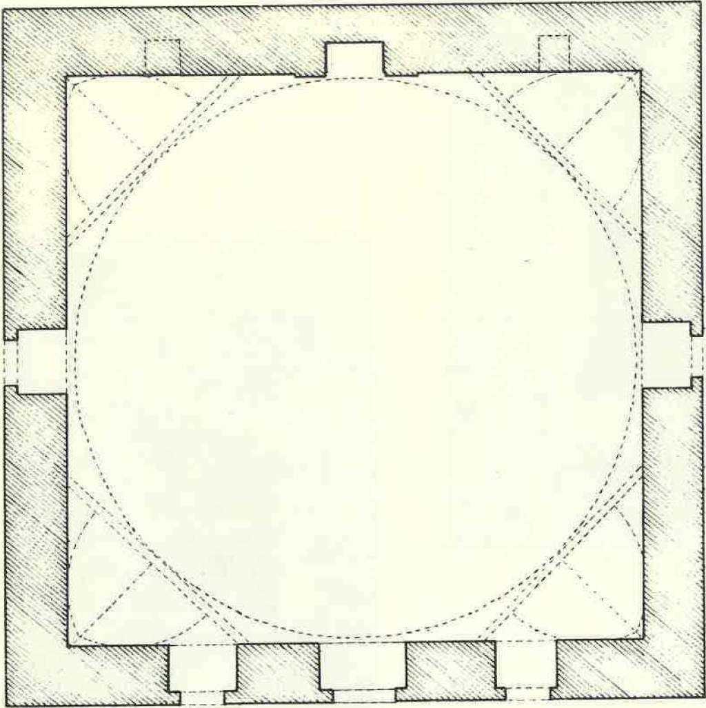
PLAN : 1 Karapınar-Kayalı Köyü yakınlarındaki Yağmıncı Obası Mescidi'nin planı.
