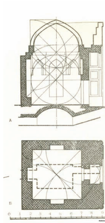
15. Hoca Ahmet Türbesi kesit ve Planı. (Nemtseva-Shvab 1979:102).
