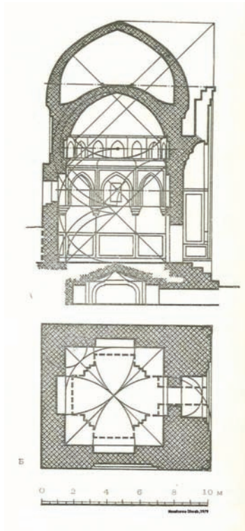
8. Emir Burunduk Tümbesi kesit ve planı. (Nemtseva-Shvab 1979:123).
