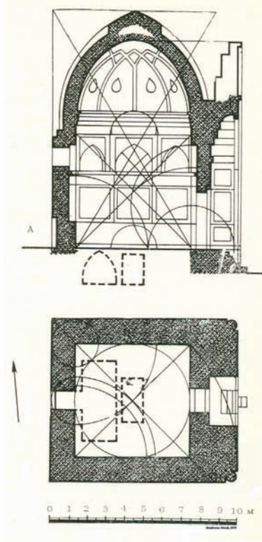
5. Şad Mülk Aka Türbesi kesit ve planı. (Nemtseva-Shvab 1979:112).
