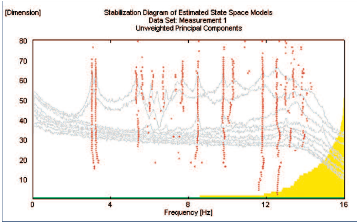
Şekil 9. Minare duvarlarında yapılan ölçümlerde stokastik altalan belirleme yöntemiyle elde edilen yığılmı değerler.
