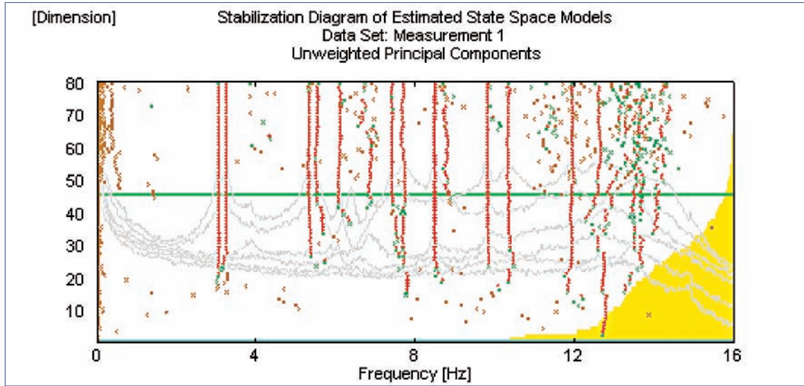
Şekil 6. Minare çekirdeğinde yapılan ölçümlerde stokastik altalan belirleme yöntemiyle elde edilen yığılmış değerler.
