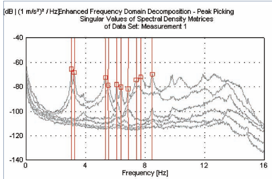
Şekil 5. Minare çekirdeğinde yapılan ölçümlerde piklerin seçilmesi yöntemiyle elde edilen tekil değerler.
