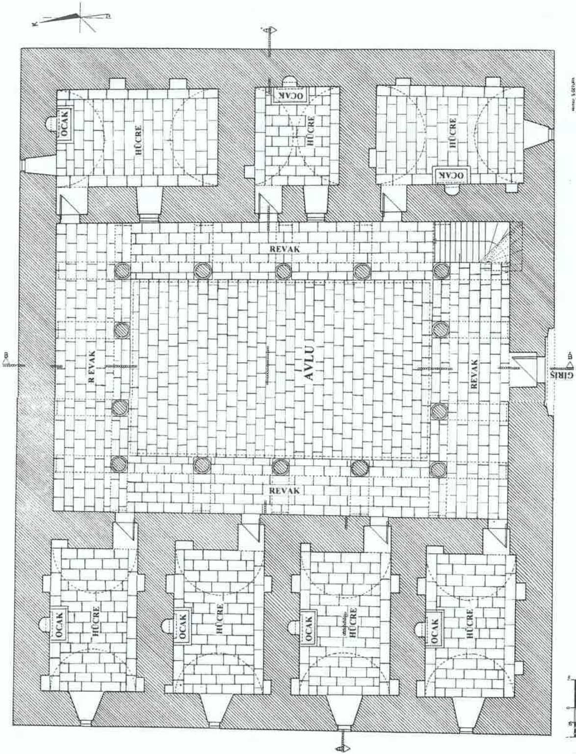
Çizim 2: Meydan Medresesi Zemin Kat Planı.
