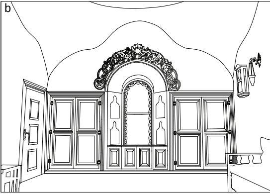
Şekil 5. Muslu Ağa Konağı tavanı (a) ve tavanla duvarın birleşmesi (b).
