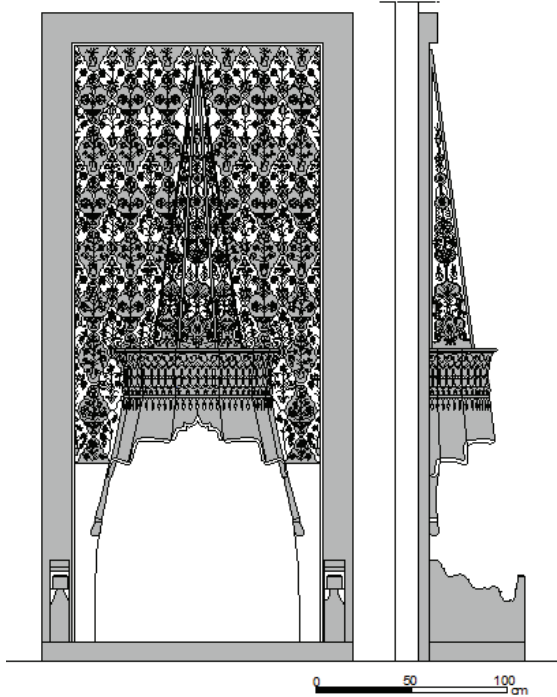
Şekil 25. Latifoğlu Konağı'nda bulunan kalemışli alçı ocak.
