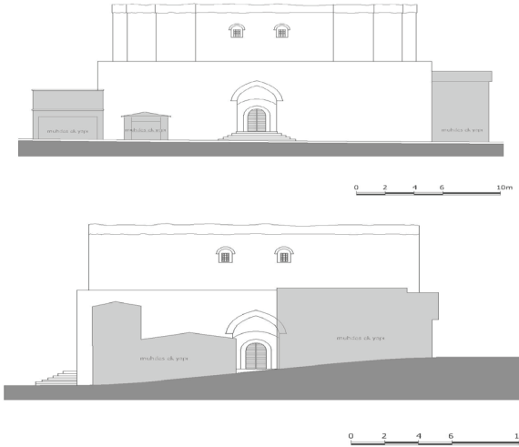
Şekil 2. Trabzon Bedesteni rolöve çizimleri devamı (Çizen, H. Emre Engin)
