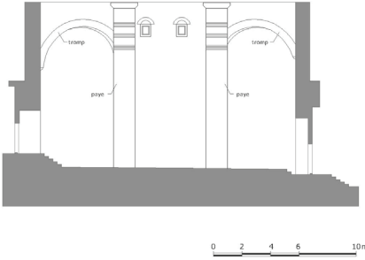
Şekil 1. Trabzon Bedesteni rolöve çizimleri (Çizen, H. Emre Engin)
