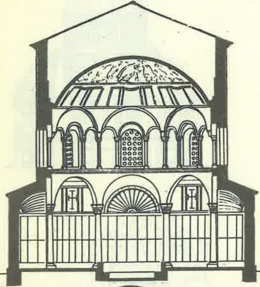
ÇİZİM : 13 Ravenna Baptisterium S. Giovanni in Fonte
