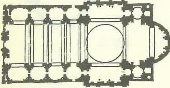
ÇİZİM : 11 Roma Gesu Kilisesi
