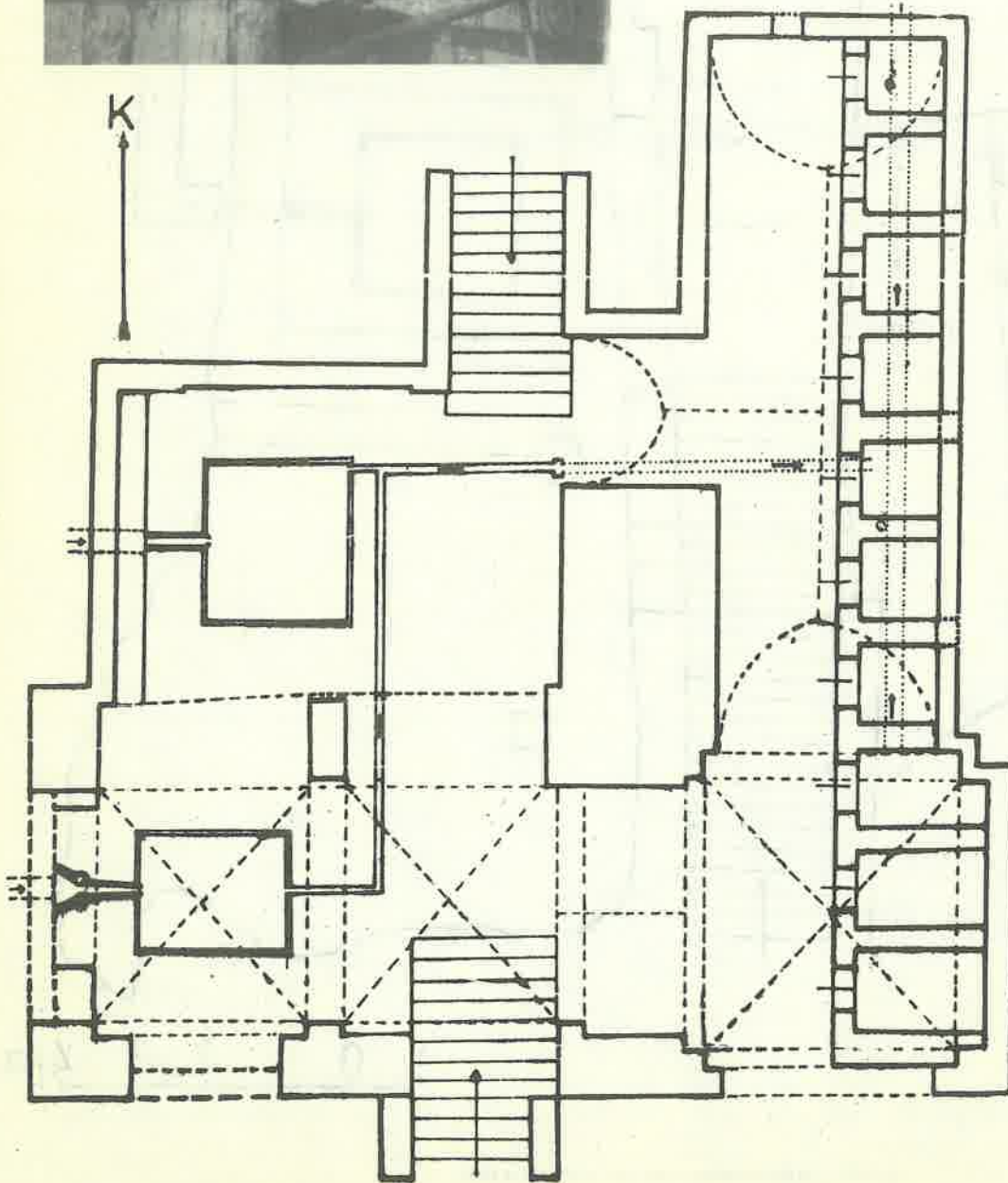
ŞEKİL: 1 Gâziantep Şeyh Fethullah Câmîi Kasteli Plânı
