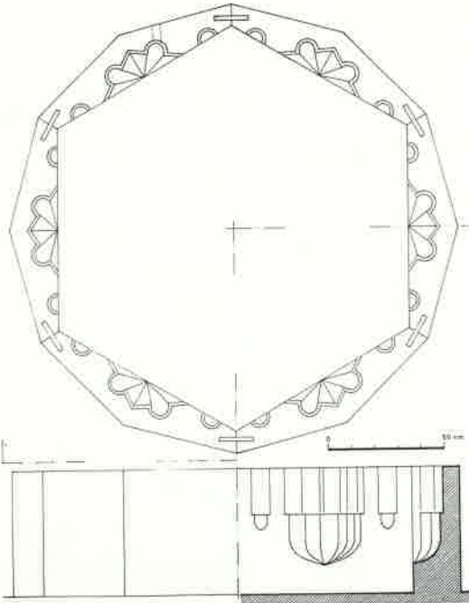
ÇİZİM: 7 Akşehir Seyyid Harun Veli Zaviyesi'nin şadırvanı
