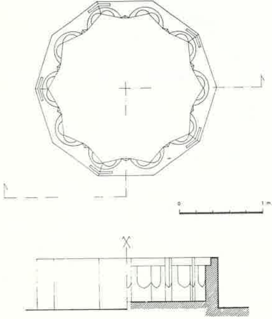
ÇİZİM: 5 Konya Türbe Hamamının kadınlar kısmı şadırvanı
