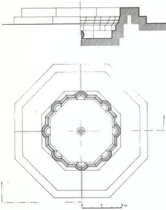
ÇİZİM: 1 Harran Ulu Camii'nin şadırvanı
