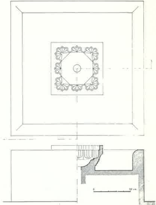
ÇİZİM: 8 Karaman Emir Süleyman Hamamı şadırvanı
