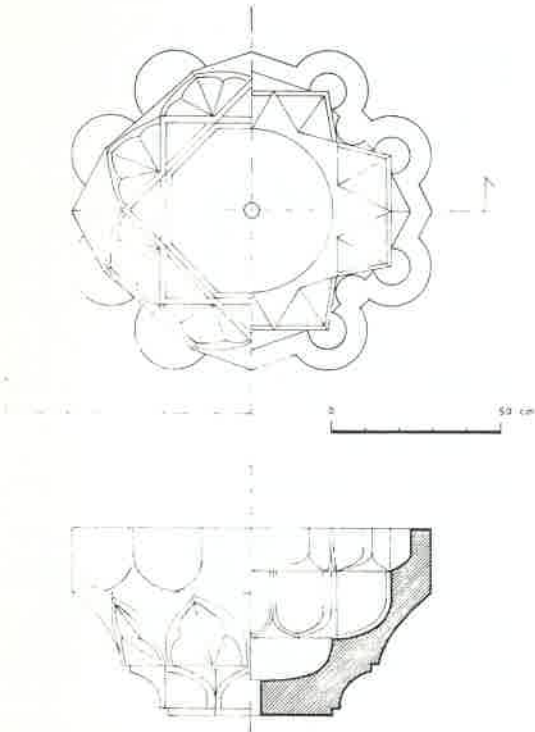
Çizim: 11 Karaman Seki Çesme Hamamının şadırvanı
