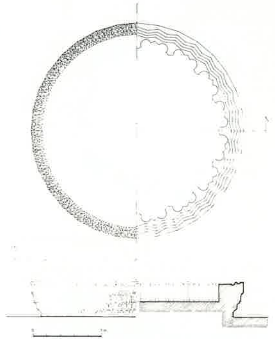
Çizim: 10 Aksaray Zincirliye Medresesi şadırvanı
