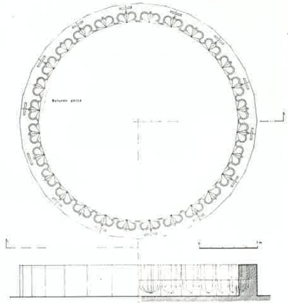
ÇİZİM: 3 Konya anonim şadırvan
