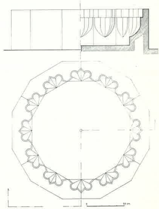
ÇİZİM: 6 Konya Türbe Hamamının erkekler kısmı şadırvanı
