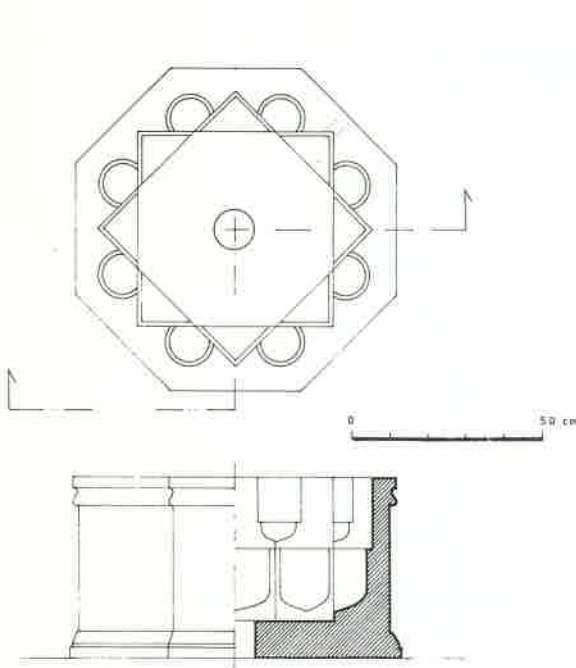
Çizim: 9 Beyşehir İsmail Ağa Hamamı (?) şadırvanı
