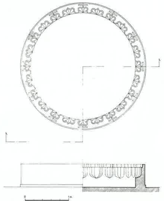
ÇİZİM: 4 Konya Türbe Hamamının (?) şadırvanı
