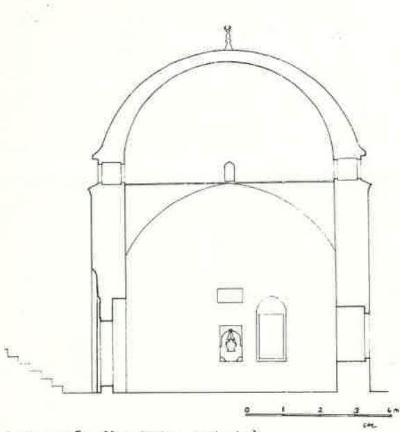
Erzurum Lale Pasa Sıbyan Mektebi A-A' Kesiti
