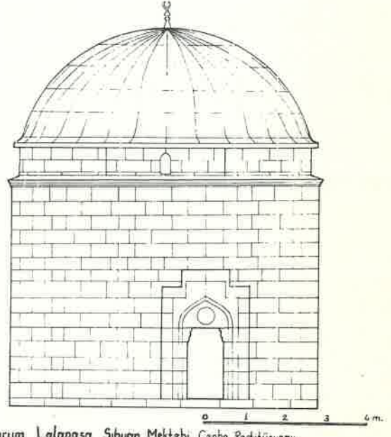
Erzurum Lale Pasa Sıbyan Mektebi Cephe Restitüsyonu
