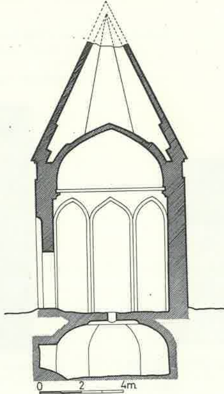
Çizim 31. Nahcivan_Yusuf bin Kuseyr (Kasir) Kumbedi. kesit
