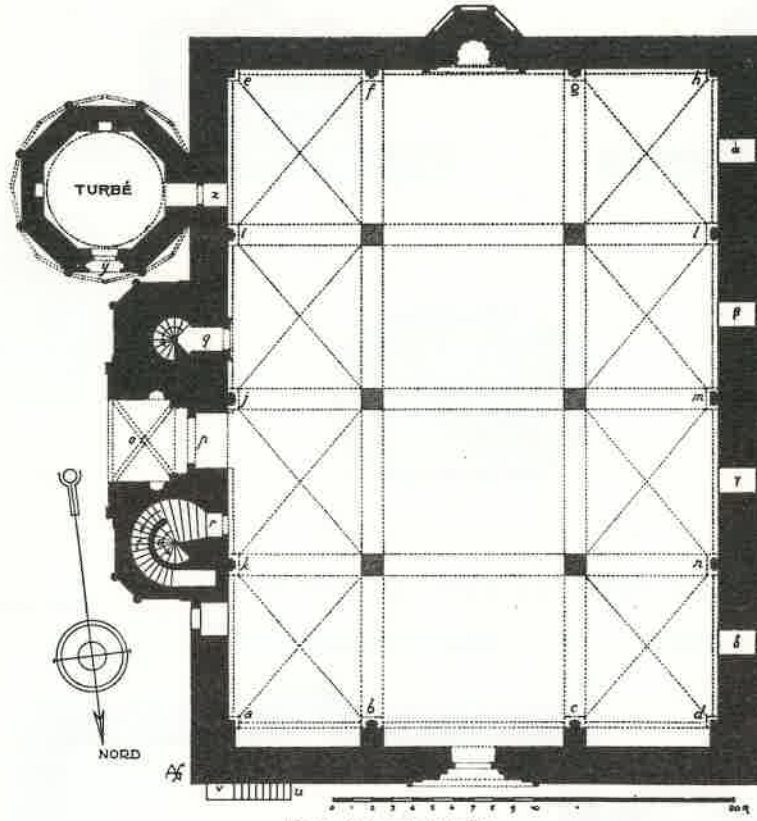
FIG. 77. — Mosquée de Sungurbey. Plan restitué.
