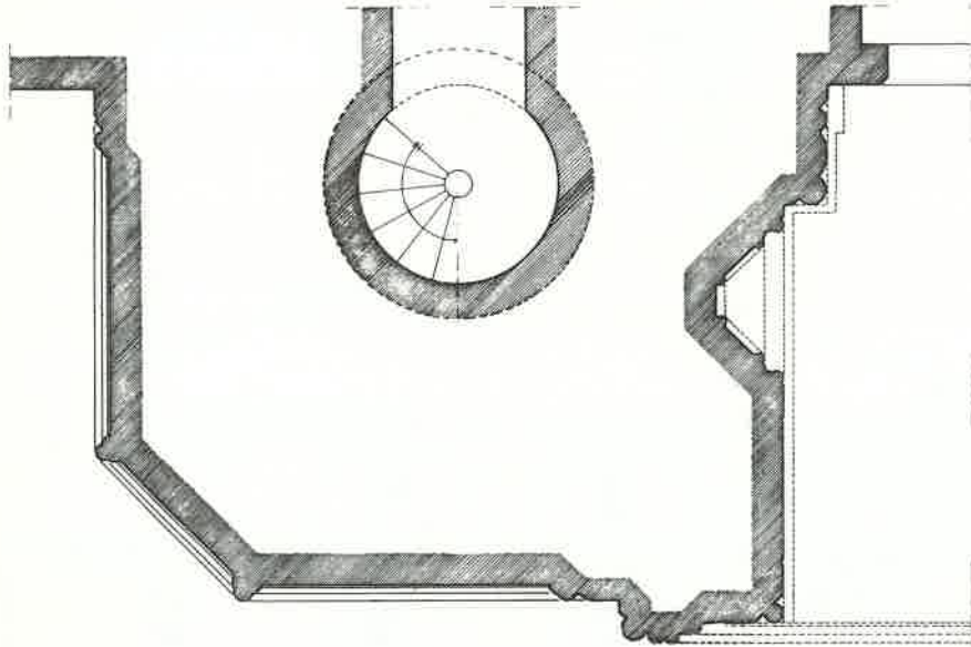
Detay - Plan Doğu Cephe Giriş Kapısı
