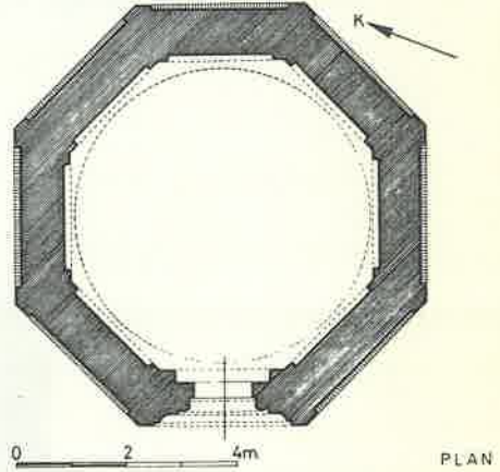
Çizim 30. Nahcivan_Yusuf bin Kuseyr (Kasir) Kumbedi. plan
