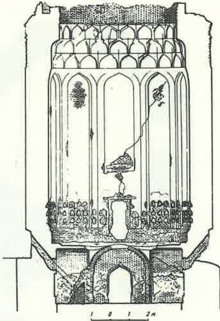
Çizim 45: Berde Kümbet, kesit
