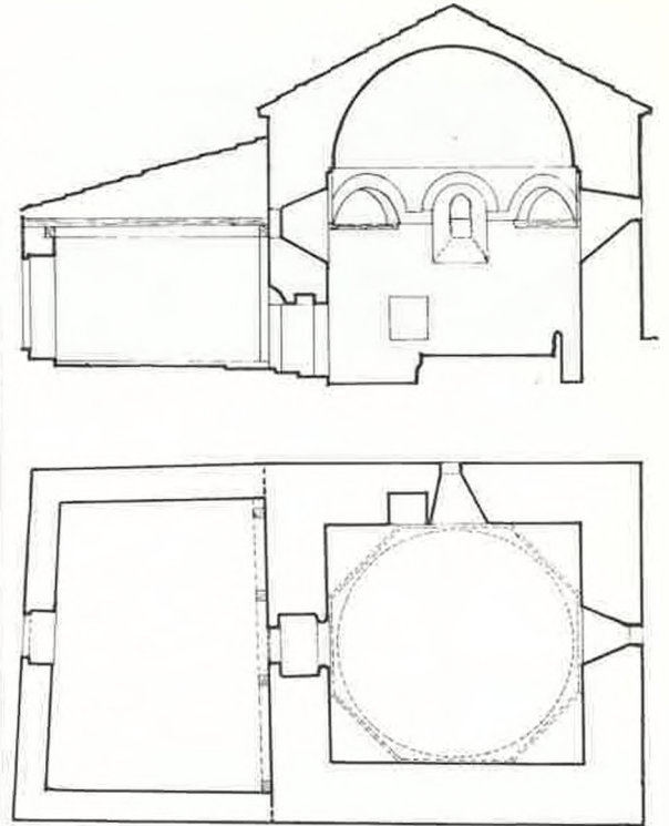
ŞEKİL: 2 Demirşeyh Türbesi plan ve kesiti
