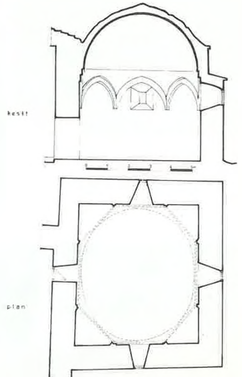
ŞEKİL: 4 Ankara-Sulakyurt Küçük Sami Köyü Türbesi plan ve kesiti
