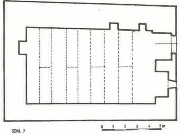
ŞEKİL: 7 Niğde İhlara Baydı Hatun Türbesi Planı
