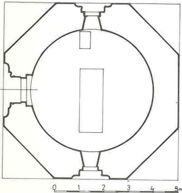
ŞEKİL: 8 Sivas Emir Ahmet Türbesi Planı
