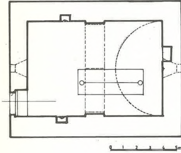
ŞEKİL: 6 Nevşehir Gülşehir Yaylacık Köyü Seyyid Ahmet Türbesi Planı
