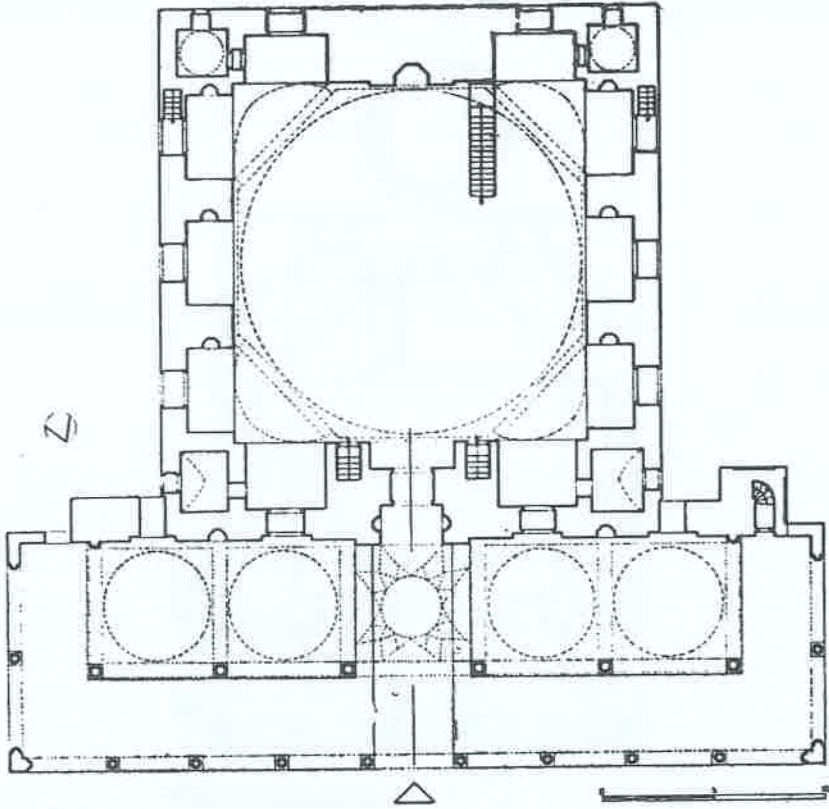
Şekil 9: Diyarbakır, Behram Paşa Camii (Sözen 1971).
