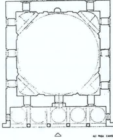
Şekil 8: Tokat, Ali Paşa Camii (Sözen 1971).
