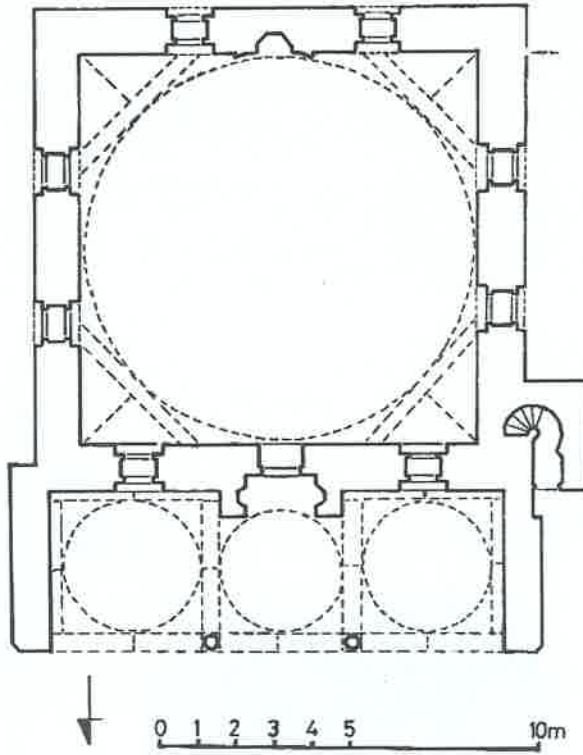
Şekil 2: Pertek, Baysungur Camii plânı (Anonim 1967'den işlenerek).
