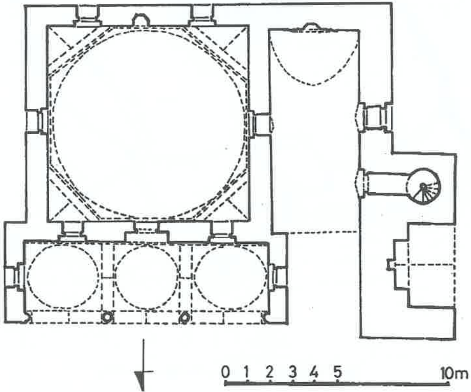
Şekil 3: Pertek, Çelebi Ali Camii plânı (Anonim 1967'den işlenerek).
