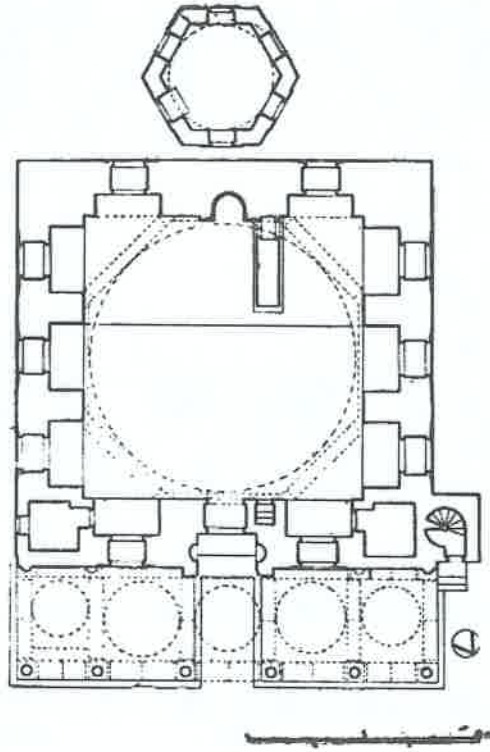
Şekil 11: Kilis, Canbolat Camii ve Türbesi (Sözen 1971).
