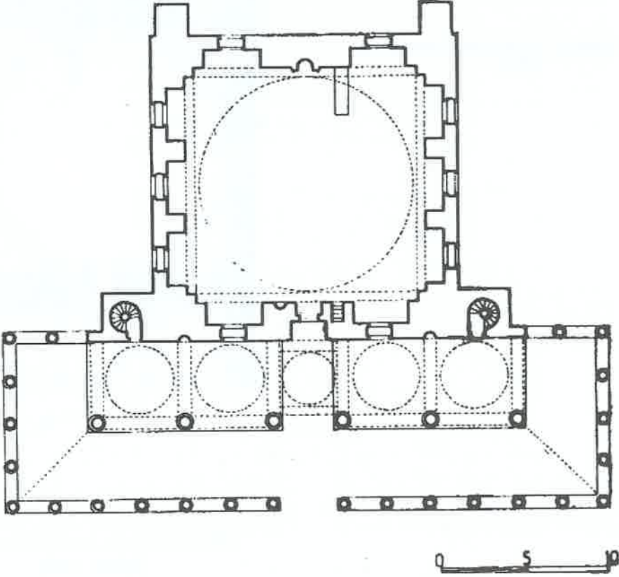
Şekil 7: Kayseri, Kurşunlu Camii plânı (Sözen 1971).
