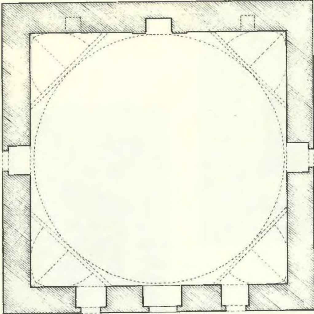
PLAN : 1 Karapınar-Kayalı Köyü yakınlarındaki Yağmapınarı Obası Mescidi'nin planı.
