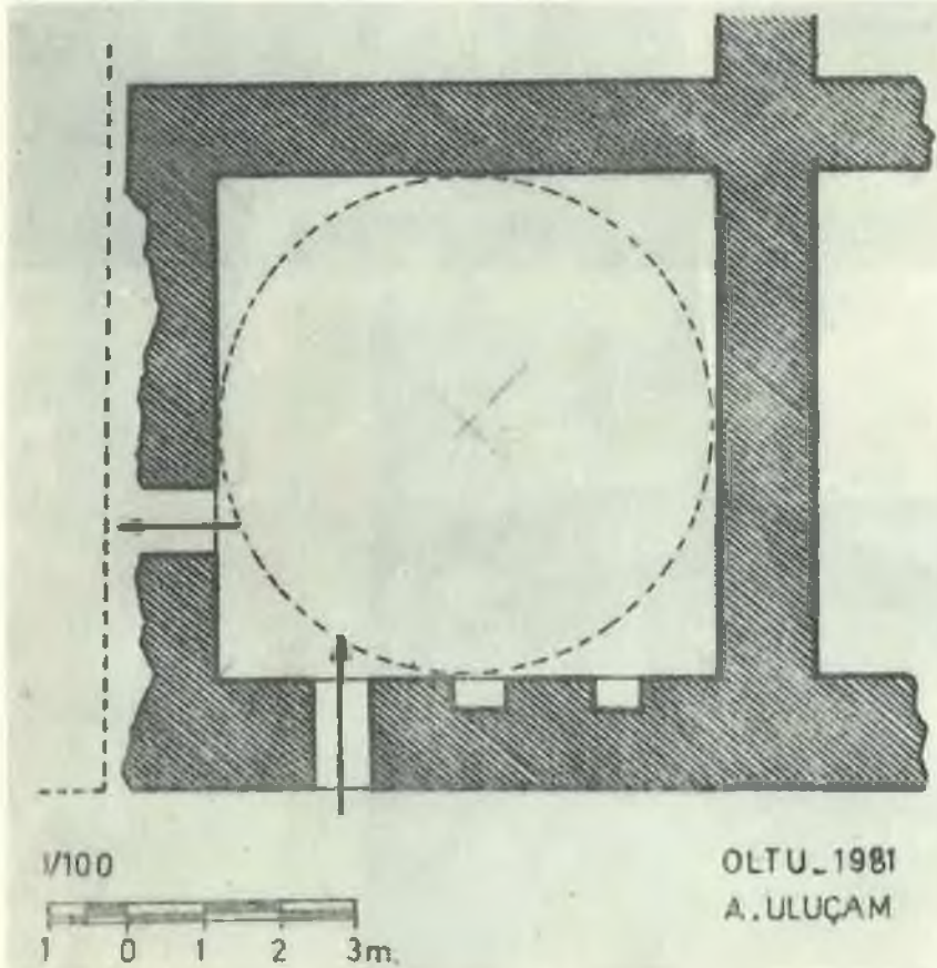
ÇİZİM: 4 Arslanpaşa Hamamı'ndan kalan kısmın piani.
